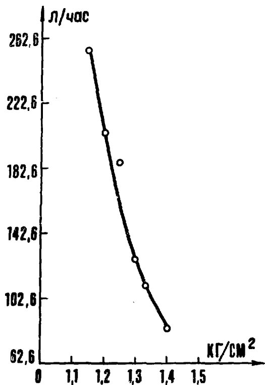
Рис. 2. Производительность компрессора по воздуху в зависимости от давления на выходе.
