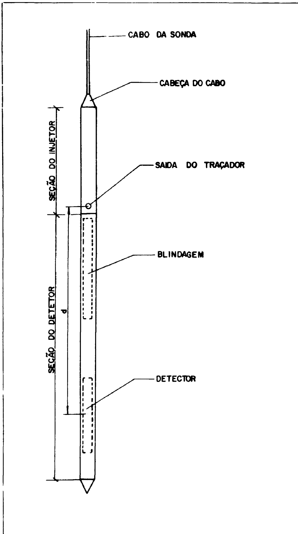
FIG. 1 ESQUEMA DE UMA Sonda INJETORA - DETECTORA, PARA A MEDIÇÃO DE FLUXOS VERTICAIS EM TUBULAÇÕES.
