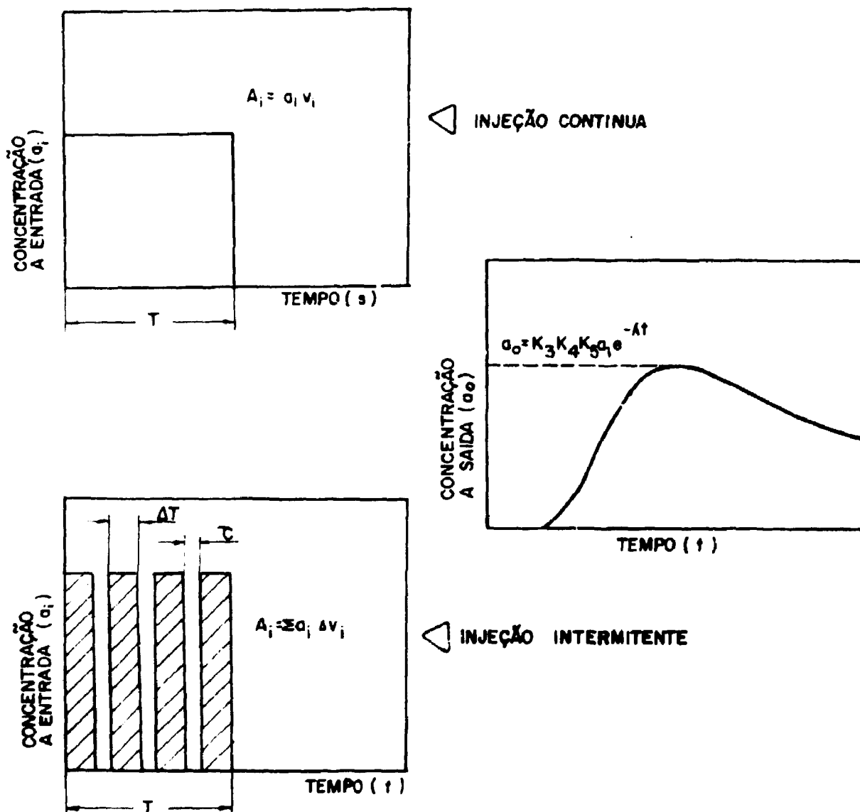
FIG. 3— CONCENTRAÇÃO DO TRAÇADOR RADIOATIVO EM FUNÇÃO DO TEMPO, A SAÍDA DO POÇO DE RECUPERAÇÃO, QUANDO A ATIVIDADE TOTAL INCORPORADA A FORMAÇÃO É IGUAL EM AMBOS OS CASOS.
