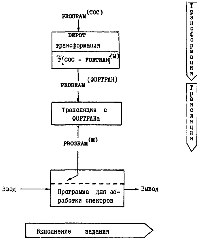
ПРИЛОЖЕНИЕ 3. Схема трансляции СОС-FOURTRAN-машинный код.
