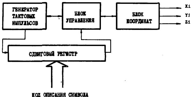
Рис. 1. Блок-схема генератора символов без буферной памяти.
