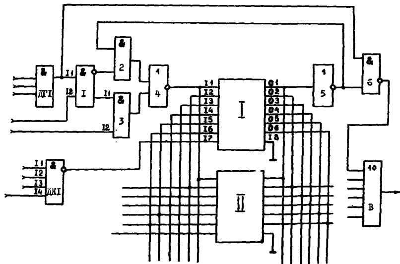
Рис. 4. Функциональная схема БЗУ на 48 слов.
