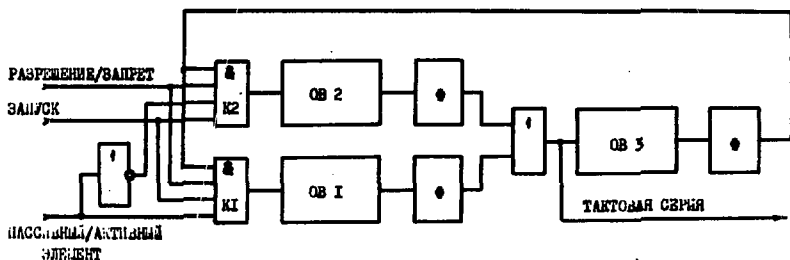
Рис. 2. Функциональная схема генератора тактовых импульсов.
