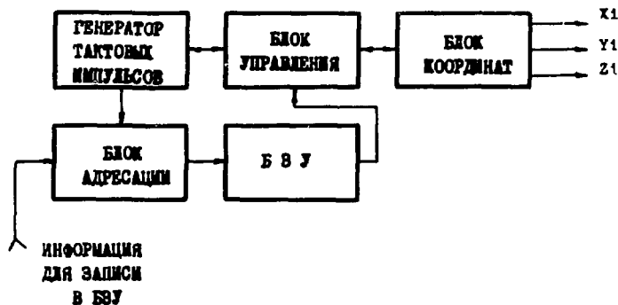
Рис. 3. Блок-схема генератора символов с буферной памятью.
