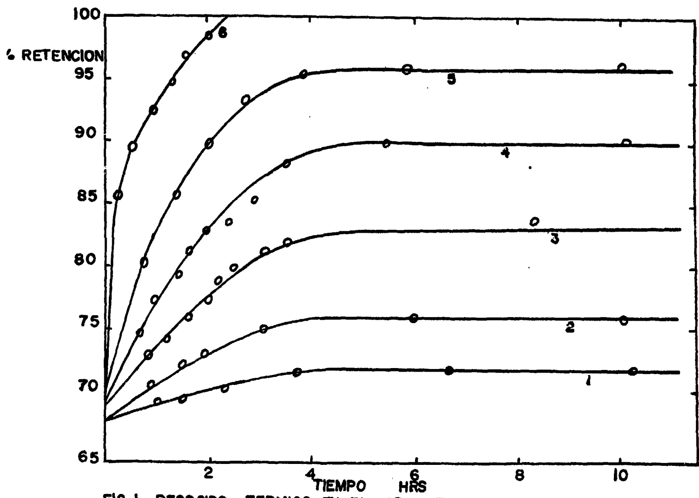
FIG.1 RECOCIDO TERMICO EN EL CROMATO DE POTASIO DESPUES DE LA REACCION NEUTRON — GAMMA CURVAS 1: 435°K, 2: 439°K, 3: 468°K, 4: 508°K, 5: 510°K, 6: 550°K,
