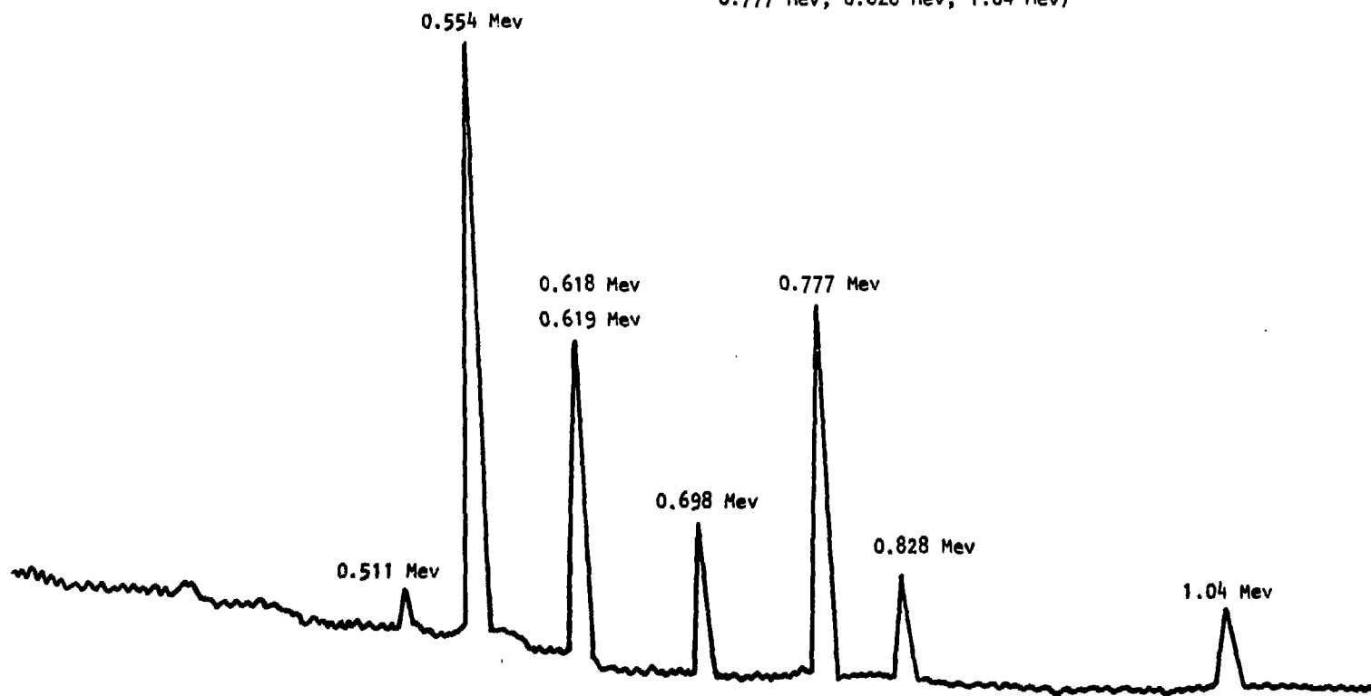
Fig. 4b) Espectro gamma obtenido en la fracción de bromatos. Espectro gamma del ^{80}\text{Br} (0.511 Mev, 0.618 Mev) Espectro gamma del ^{82}\text{Br} (0.554 Mev, 0.619 Mev, 0.698 Mev, 0.777 Mev, 0.828 Mev, 1.04 Mev)
