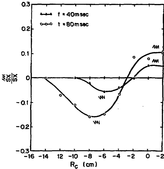
第13図 ケースCにおける散X線成分の R_C 依存性
