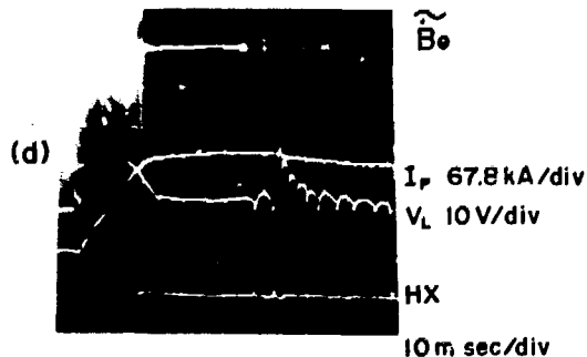
第7図 代表的放電特性のオシログラム写真。ここで \tilde{B}_0 はポロイダル磁場の微分波形、 I_P はプラズマ電流、 V_L は1ターンの電圧、HXは硬X線によるNaI出力を示す。
