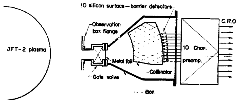
第1図 内部振動測定器の構造
