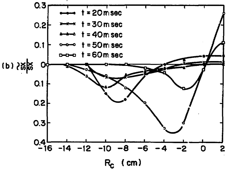
第11図 ケースAにおけるポロイダル磁場の振動成分の位相変化(a)および軟X線の振動成分の R_0 依存性
