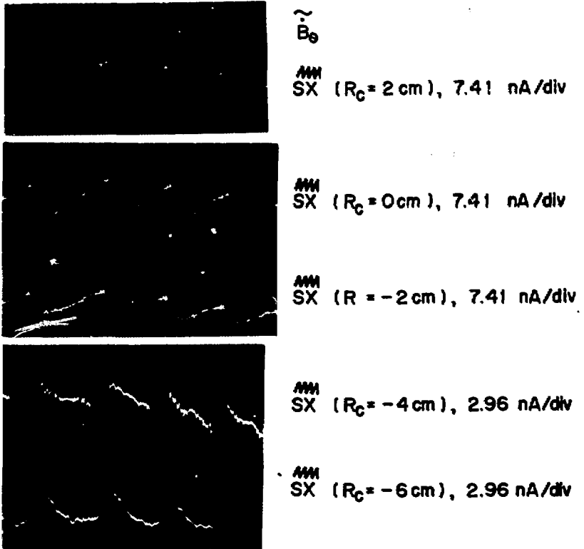
第14図 内部スパイク振動の拡大図(ケースC t = 80 \text{ msec} ) 掃引時間 : 1 msec/div
