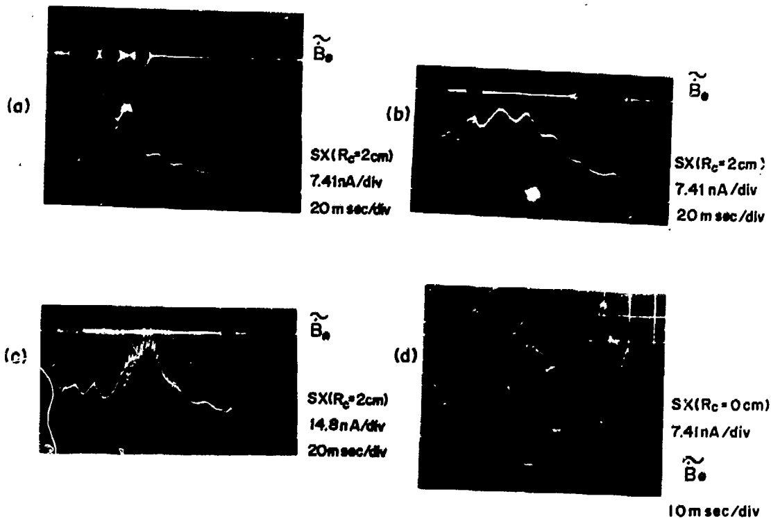
第9図 各ケースにおけるSSD出力の時間変化のオシログラム写真
