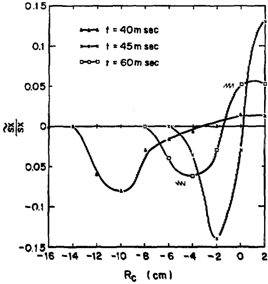
第12図 ケースBにおける散X線成分の R_C 依存性
