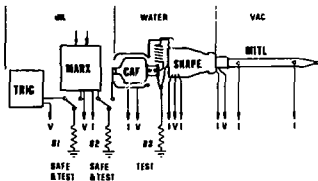
Fig. 12. PBFA-I Divertor Test.
