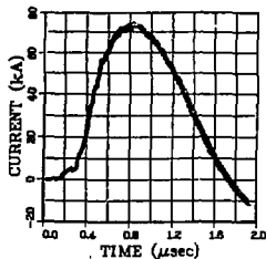
Fig. 13. Marx Generator Output Data.
