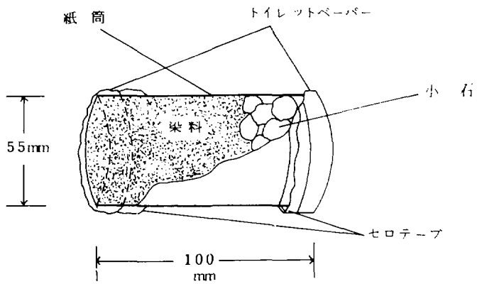
第2図 粉末染料投入ケース
