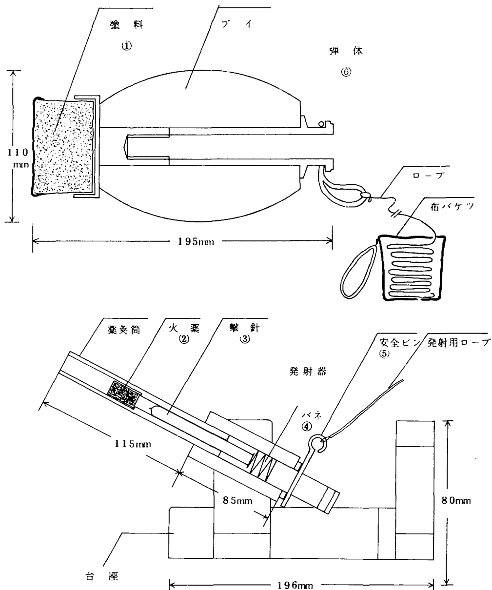
第3図 染料投入器
