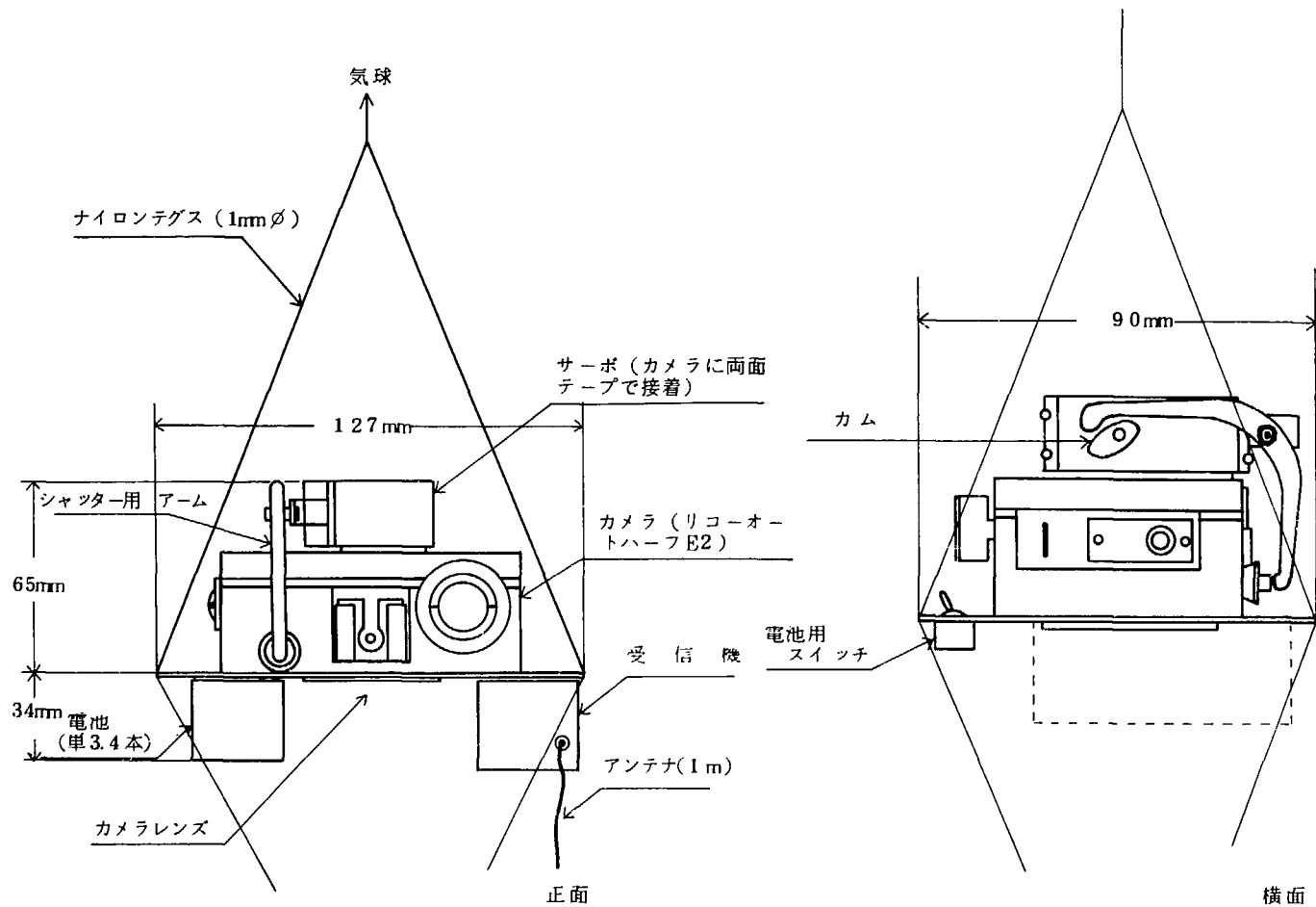
第5図 撮影カメラ及びリモコンメカニズム
