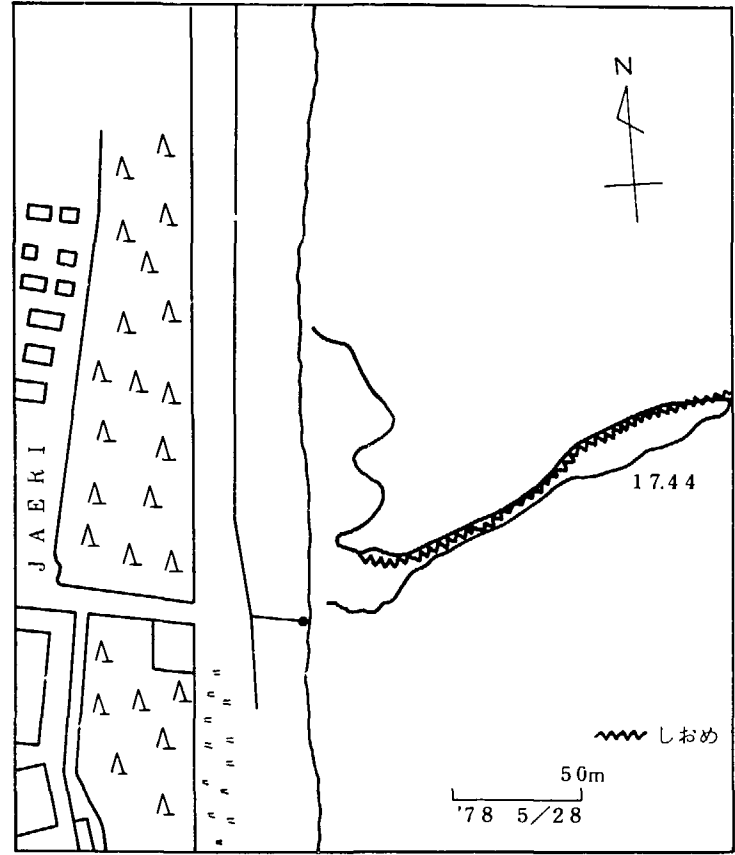
第9図(c) 染料拡散の例(4) 1978年5月28日 しおめ付近の染料の流動と拡散 17時44分
