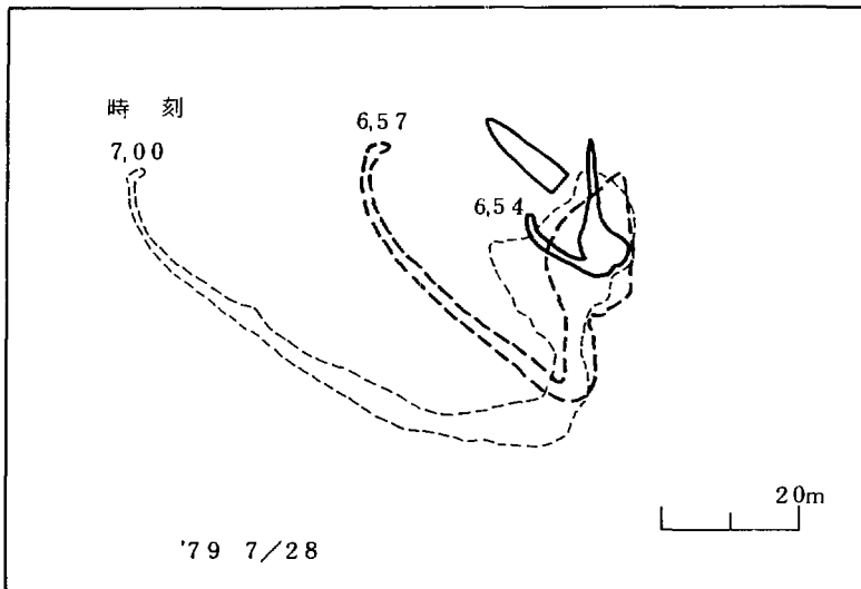
第20図 沖合での染料拡散の例(15) 1979年7月28日 鉛直シヤのある場合
