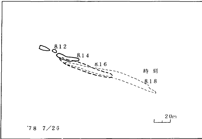
第15図 沖合での染料拡散の例(10) 1978年7月26日 強い表層流のある場合
