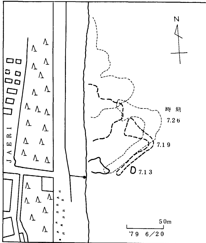
第10図 染料拡散の例(5) 1979年6月20日 沿岸流と沖合流が同じ方向の場合
