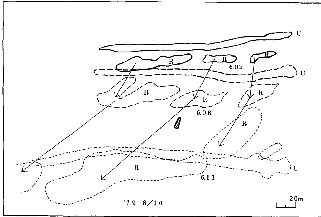
第22図 沖合での染料拡散の例(17) 1979年8月10日 沢山の染料雲の拡散の例
