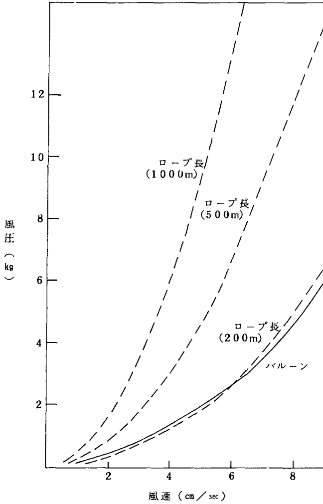
第4図 気球及び係留索の受ける風圧と風速の関係
