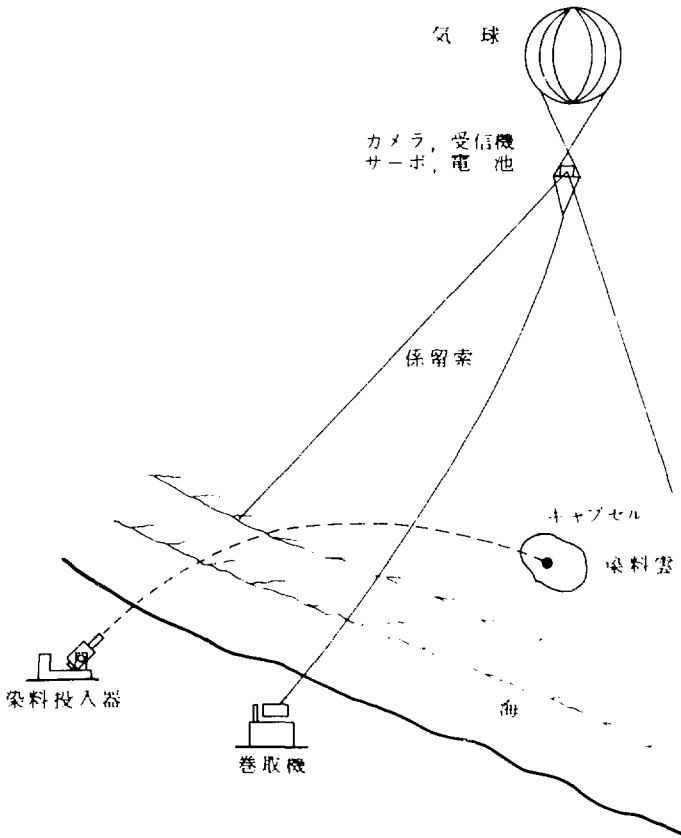
第1図 沿岸染料拡散実験配置図
