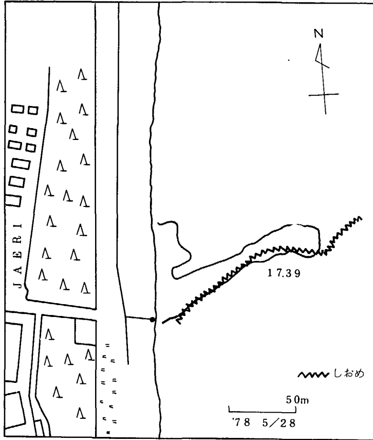
第9図(b) 染料拡散の例(4) 1978年5月28日 しおめ付近の染料の流動と拡散 17時39分
