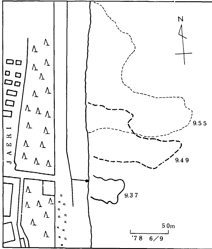
第8図 染料拡散の例(3) 1978年6月9日 沿岸流, 離岸流共に強い。
