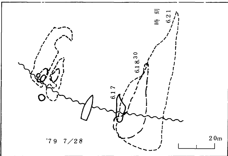
第18図 沖しおめ付近での染料拡散の例(13) 1979年7月28日
