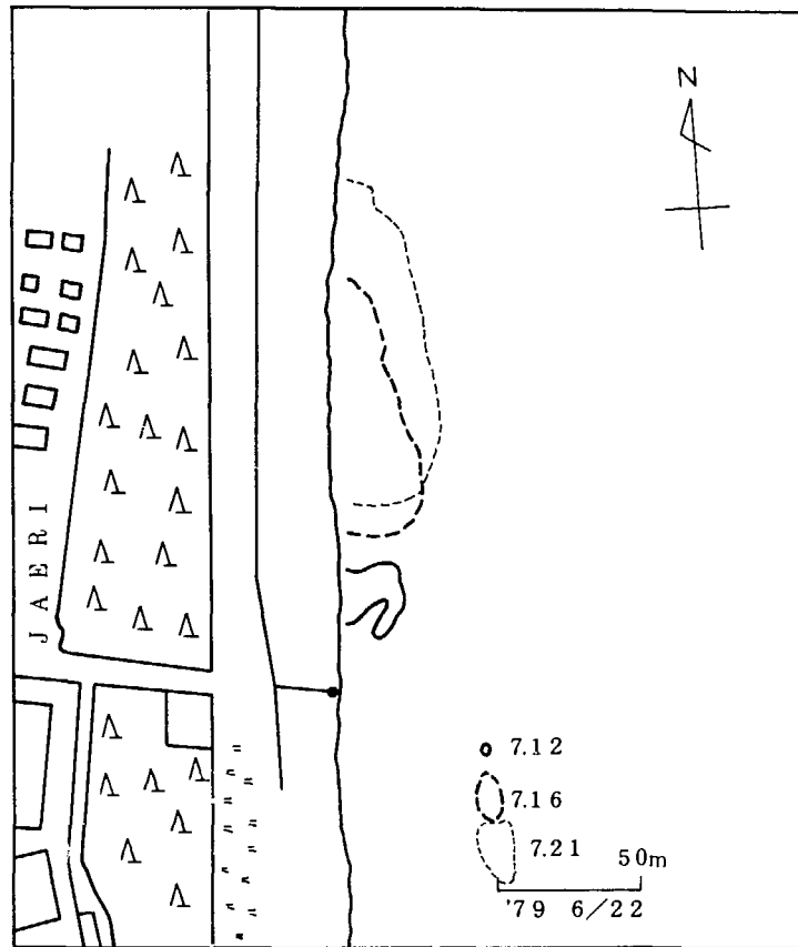
第11図 染料拡散の例(6) 1979年6月22日 沿岸流と沖合流の方向が逆の場合
