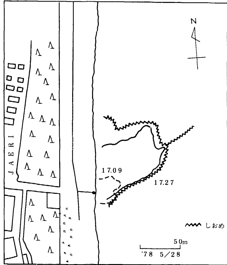
第9図(a) 染料拡散の例(4) 1978年5月28日 しおめ付近の染料の流動と拡散 17時09分~17時27分
