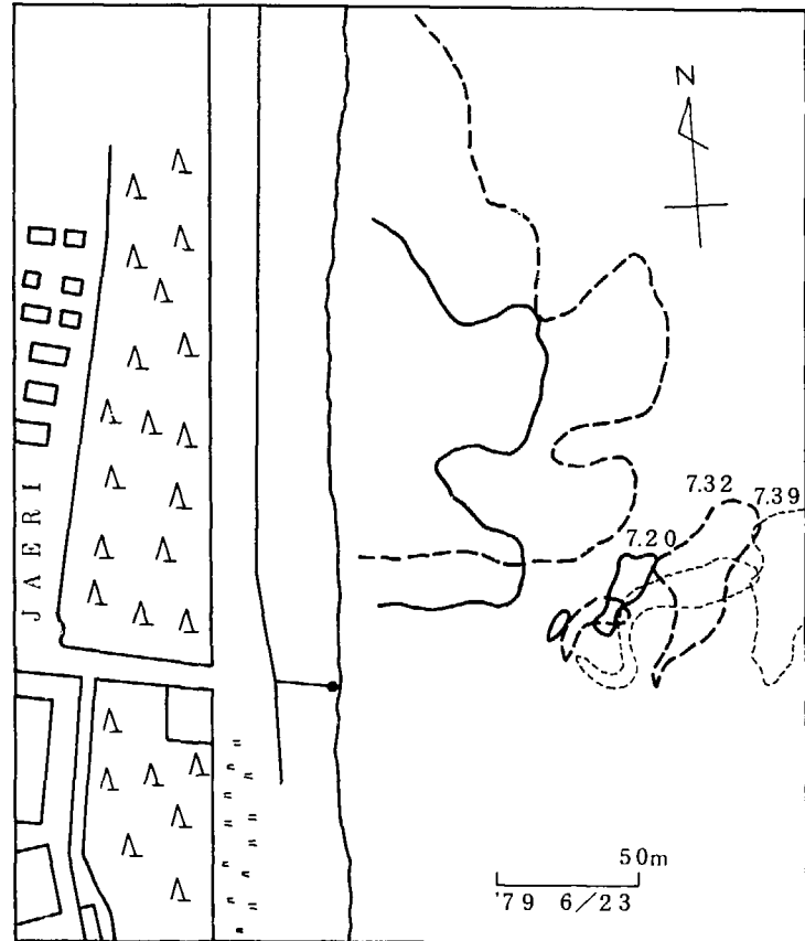
第13図 染料拡散の例(8) 1979年6月23日 沿岸流がほとんど停止し、中合表層流が沖方向に流れる場合
