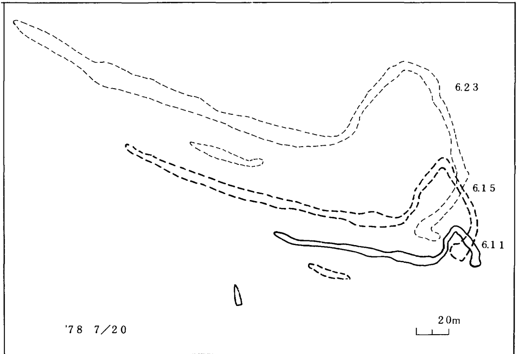
第16図 沖合での染料拡散の例(11) 1978年7月20日 流れの方向が表層・中層・底層で異なる場合
