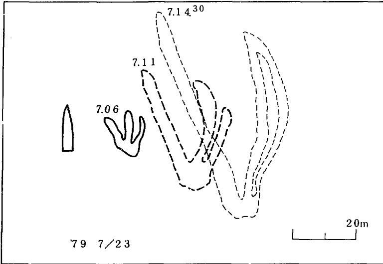
第19図 沖合での染料拡散の例(14) 1979年7月23日 鉛直シヤのある場合
