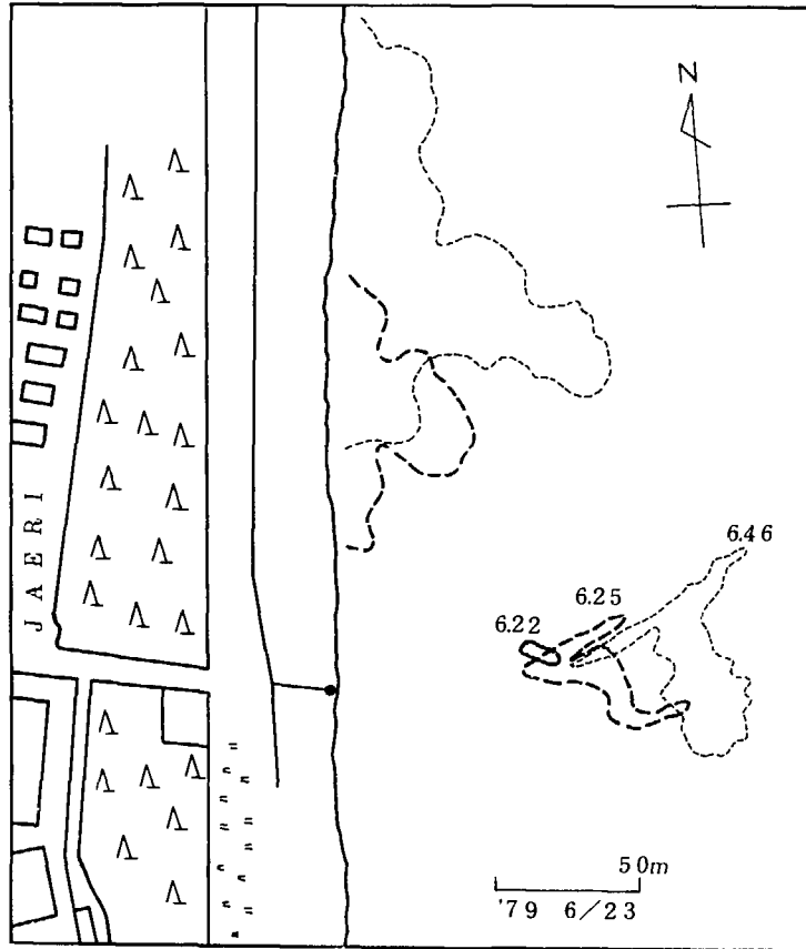
第12図 染料拡散の例(7) 1979年6月23日 沿岸流が北に沖合表層流が沖方向に流れる場合
