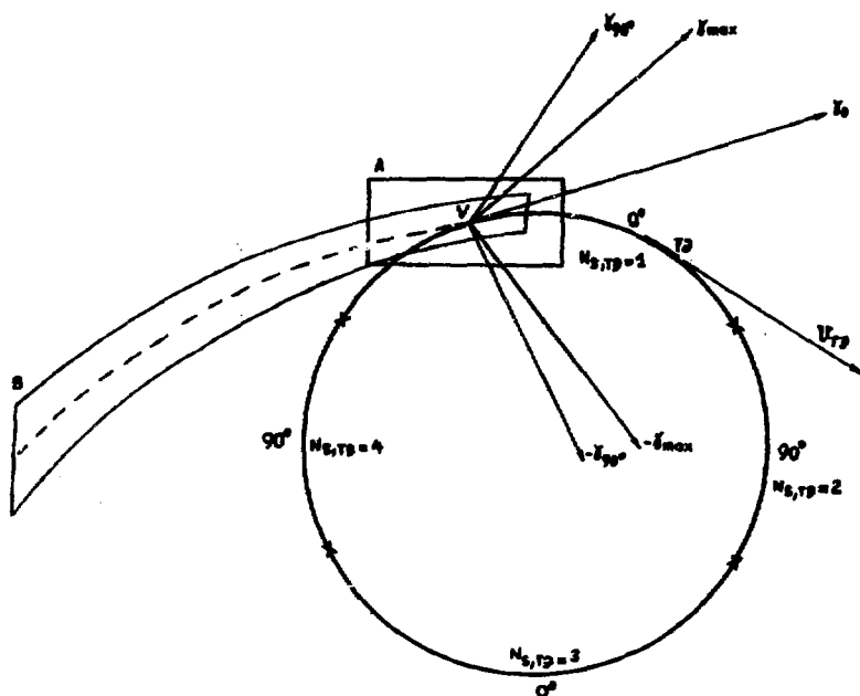
Рис. 1. V - вершина события; A - зона вершины; B - зона пучкового трека; N_{с,тэ} - порядковые номера сегментов кругового трека, порожденного трех-элементом ТУ и вершиной V ; \gamma_{90}^0 - предельный угол трека, допускающий использование моды сканирования 0^0 ; \gamma_{max} - предельный угол выхода вторичных треков из вершины; \gamma_0 - угол касательной к круговому треку в точке вершины.
