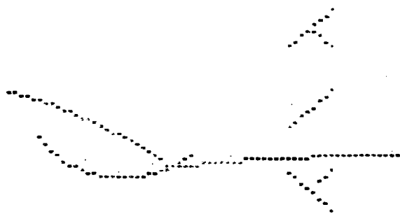
Рис. 2б. Данные рисунка 2а после префильтра. Условия предварительной фильтрации: 1) Y_{\max} = 45^{\circ} , 2) дескриптор вершины осадки: а) признак выхода вторичных треков под большим углом (больше Y_{90} ) и б) признак наличия вторичных треков в задней полушаре.
