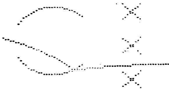
Рис. 2а. Графическая распечатка результатов математического моделирования процесса сканирования (мода 0^{\circ} ) и последующего преобразования их в трек-элементе. Плечи реперных крестов под углом \pm 45^{\circ} , угол выхода прямого трека 35^{\circ} , угол выхода кругового трека 30^{\circ} .
