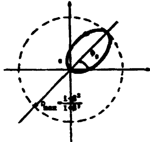
Fig. 2a: \beta = 0
