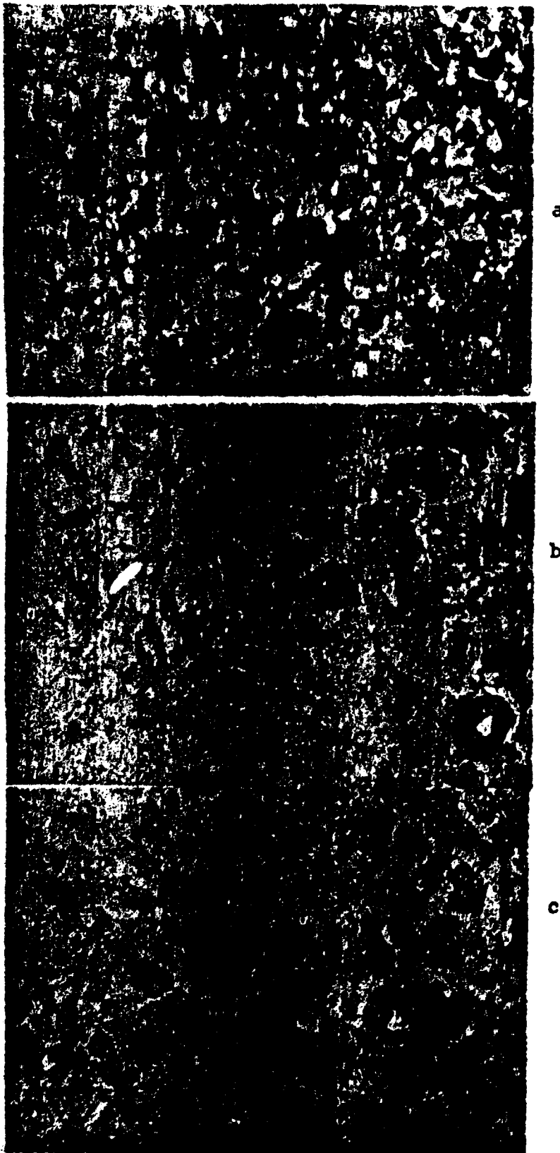
Fig. 4 - Influência do teor de Nb nas estruturas fundidas e normalizadas a 900°C - 2h; do aço ABNT 4140; a) normal; b) 0,1% Nb e 0% Mo; c) 0,2% Nb e 0% Mo. Ataque: Nital - 200x.
