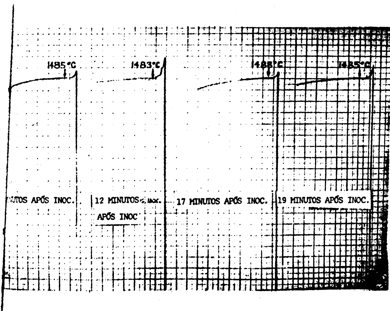
Fig. 2 - Curvas de esfriamento do aço ABNT 4140 modificado (0,1%Nb + 0,1%Mo) após vários tempos de inoculação. Verifica-se o patamar de solidificação não se alterou sensivelmente.
