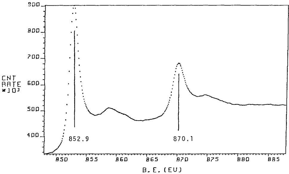
Fig. 56 Ni 2p XPS spectrum of Ni et .
