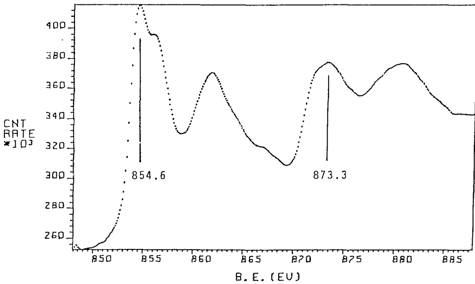
Fig. 58 Ni 2 p XPS spectrum of NiO.
