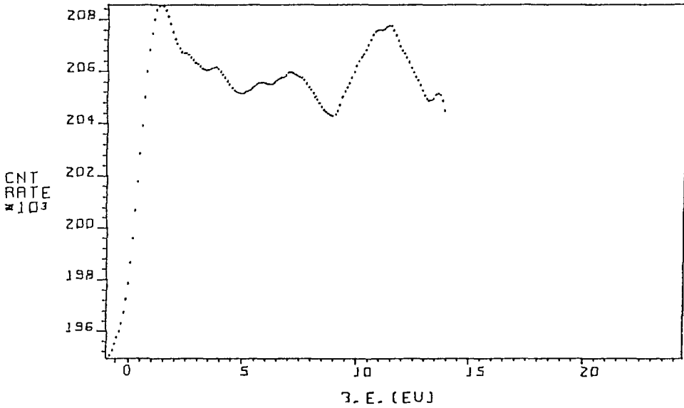
Fig. 26 Valence-band spectrum of Ti et .
