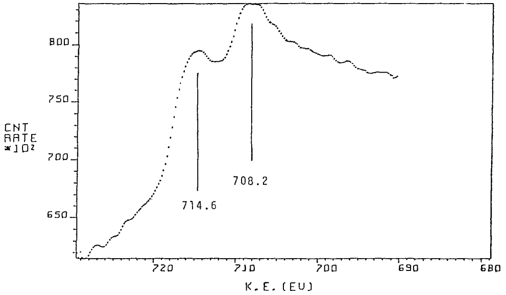
Fig. 55 L 3 VV XAES spectrum of Ni fl .
