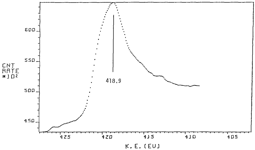
Fig. 24 L 3 M 2,3 V XAES spectrum of Ti fl .
