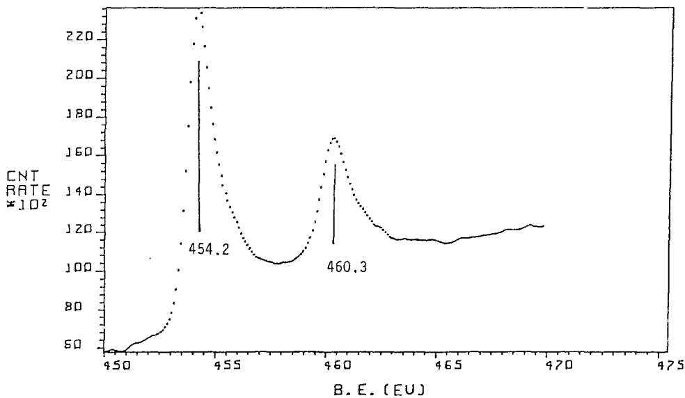
Fig. 20 Ti 2p XPS spectrum of Ti fl .
