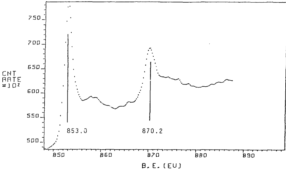
Fig. 51 Ni 2p XPS spectrum of Ni fz .
