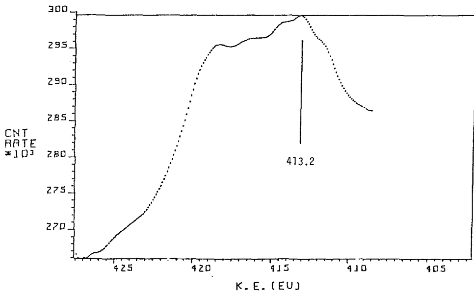
Fig. 32 L 3 M 2,3 V XAES spectrum of TiO 2 .
