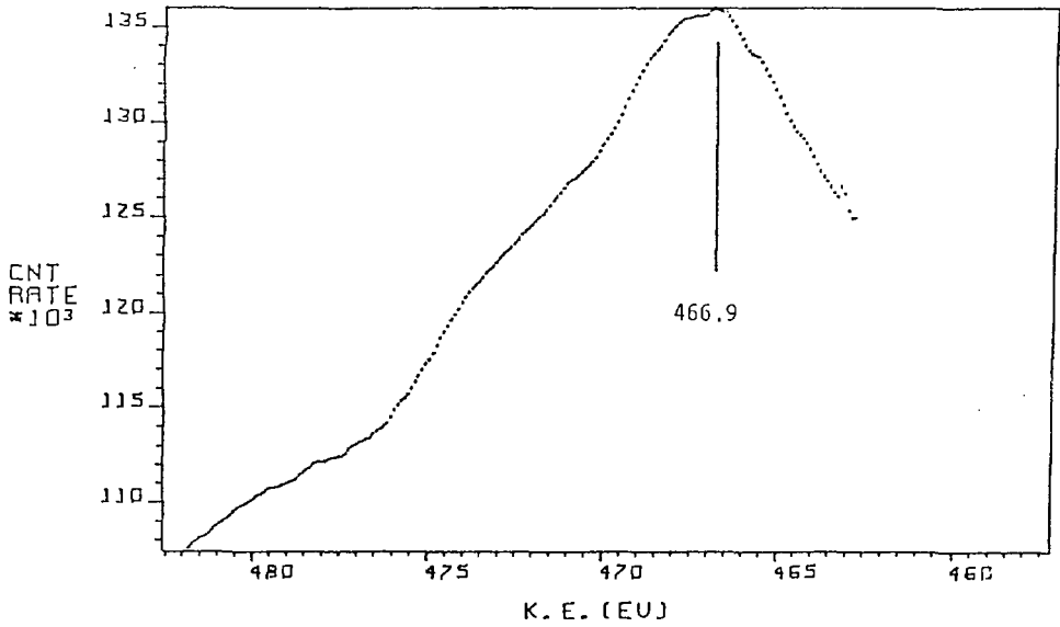
Fig. 48 L 3 M 2,3 M 2,3 XAES spectrum of V 2 O 5 .
