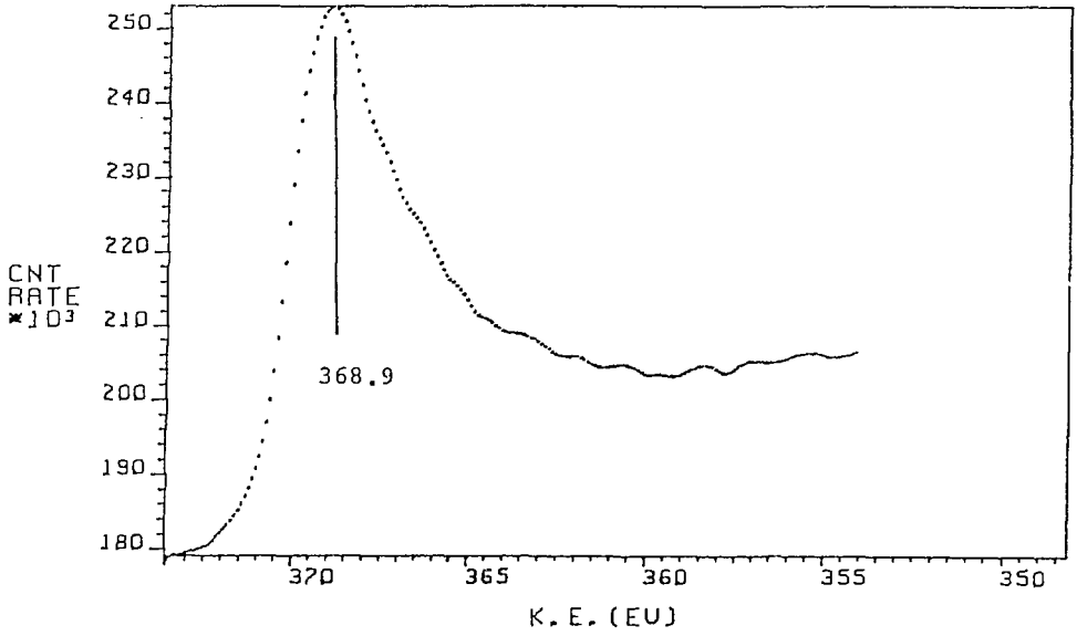
Fig. 11 L 2,3 M 2,3 V XAES spectrum of Sc et.
