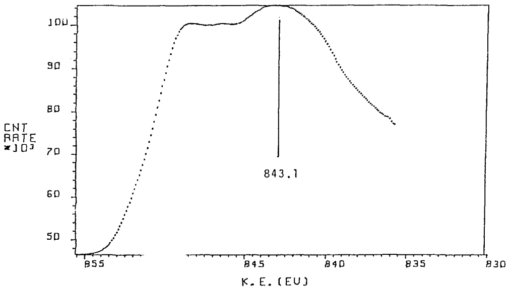
Fig. 60 L 2 VV XAES spectrum of NiO.
