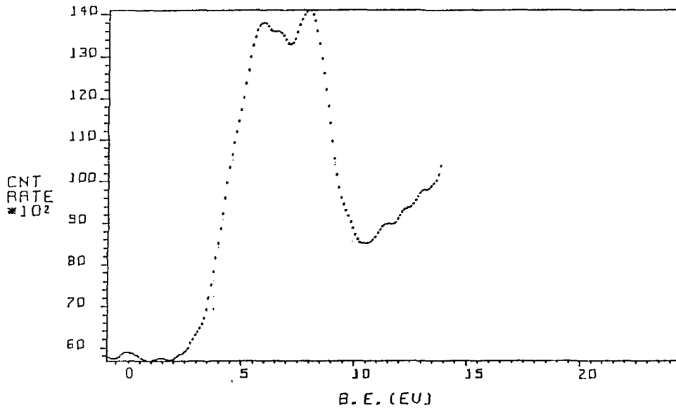
Fig. 31 Valence-band spectrum of TiO 2 .
