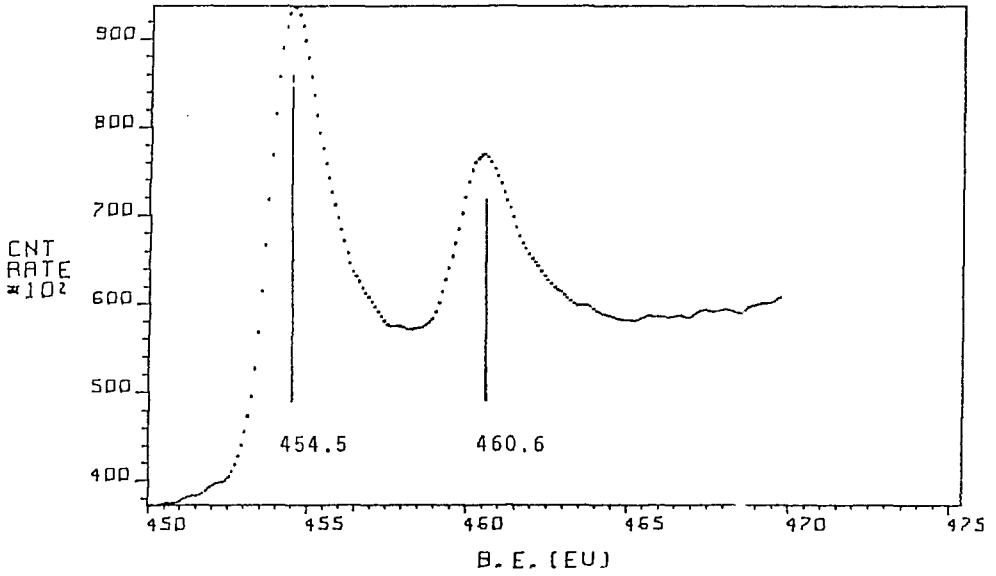
Fig. 25 Ti 2p XPS spectrum of Ti et .
