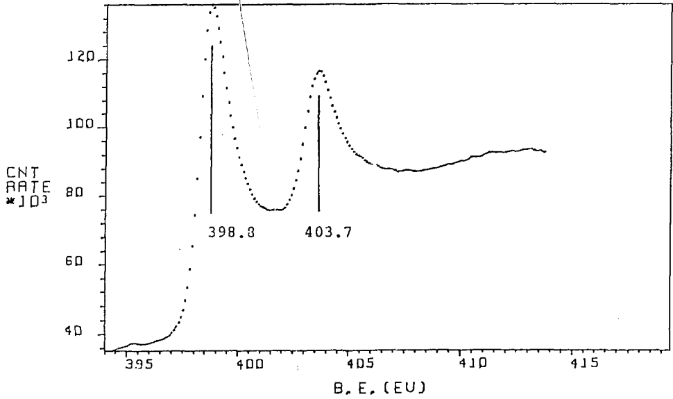
Fig. 9 Sc 2p XPS spectrum of Sc et .
