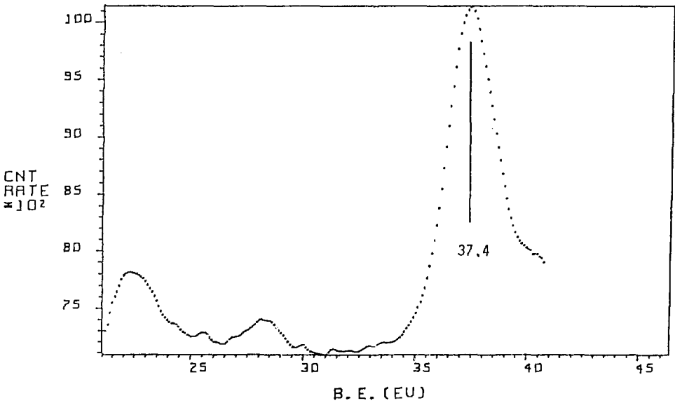
Fig. 30 Ti3p XPS spectrum of TiO 2 .
