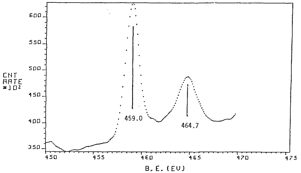
Fig. 28 Ti_{2p} XPS spectrum of TiO_2 .
