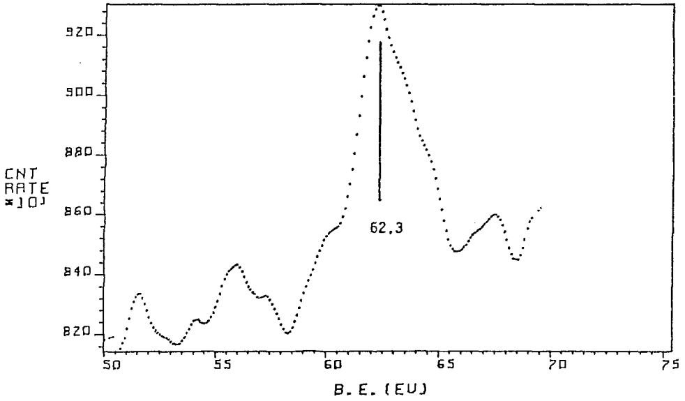
Fig. 29 Ti3s XPS spectrum of TiO 2 .
