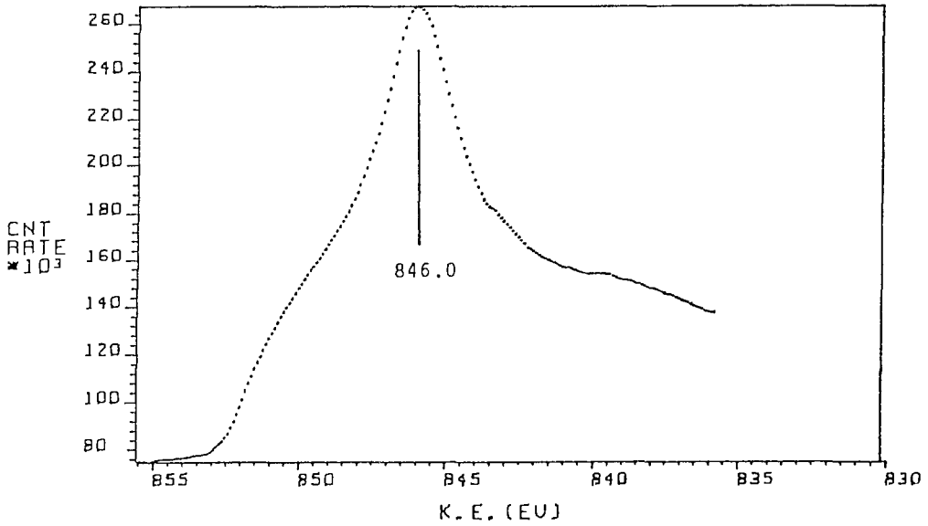
Fig. 57 L 3 VV XAES spectrum of Ni et .
