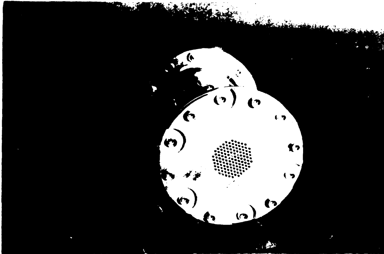
Fig. 7 - Foto do primeiro modelo do propulsor iônico.
