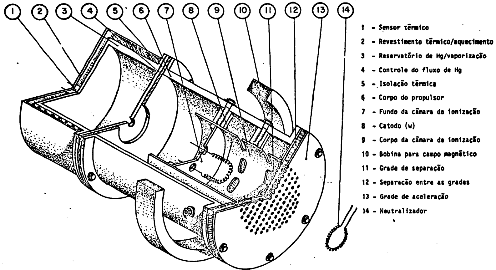
Fig. 6 - Corte do primeiro modelo do propulsor iônico
