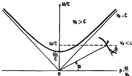
Fig. 16 - Brillouin diagram
