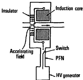
Fig. 10- Linear induction accelerator module
