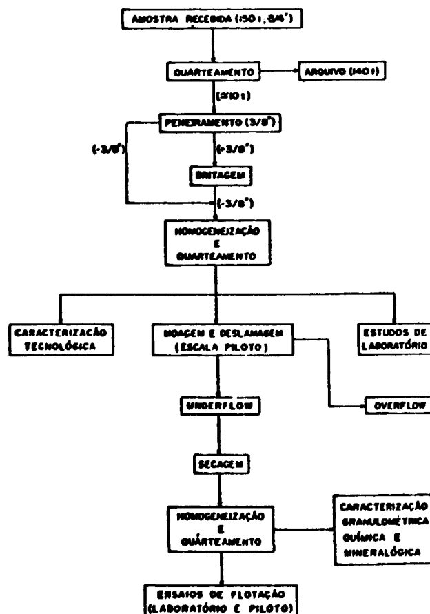
FIGURA 1 - Fluxograma utilizado na preparação das amostras
