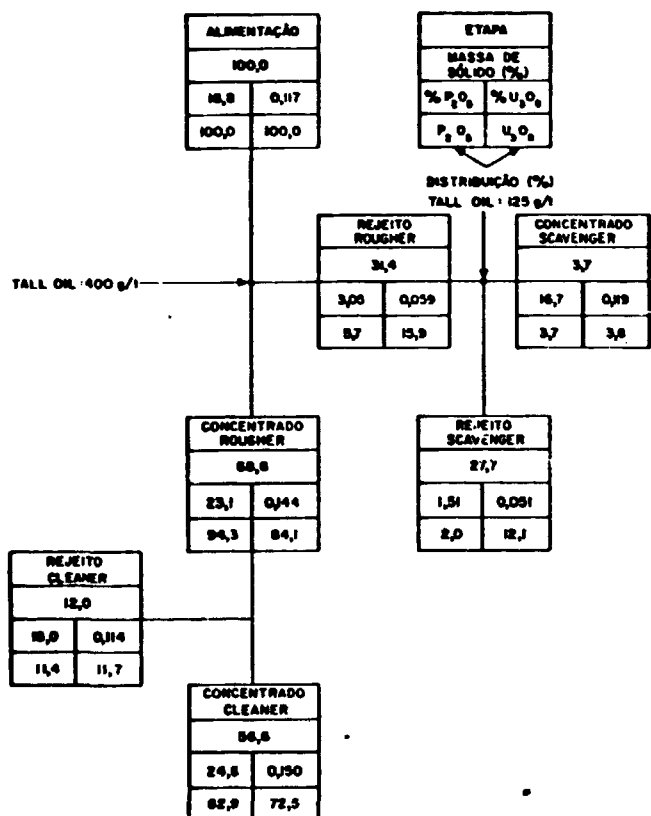
FIGURA 17 - Balanço de massa e metalúrgico sem adição estagiada de "Tall Oil"
