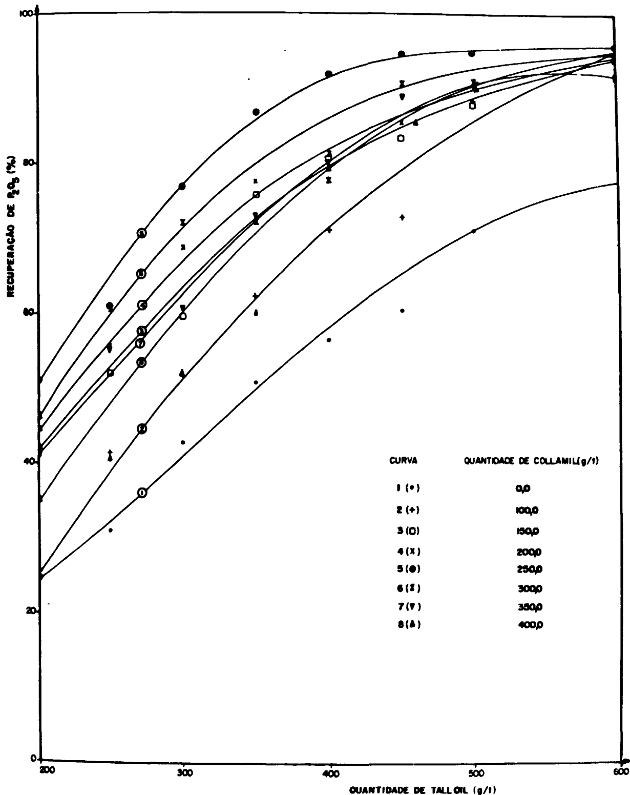
Figura 2 - Efeito da quantidade de tall oil, sobre a recuperação de P_2O_5 , para diferentes quantidades de collamil
