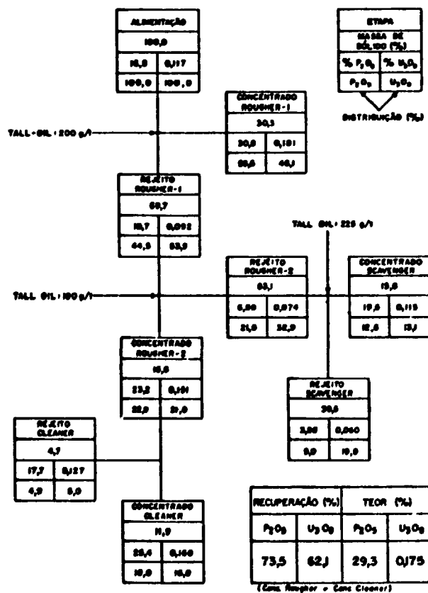
FIGURA 19 - Balanço de massa e metalúrgico com adição estagiada de "Tall Oil"
