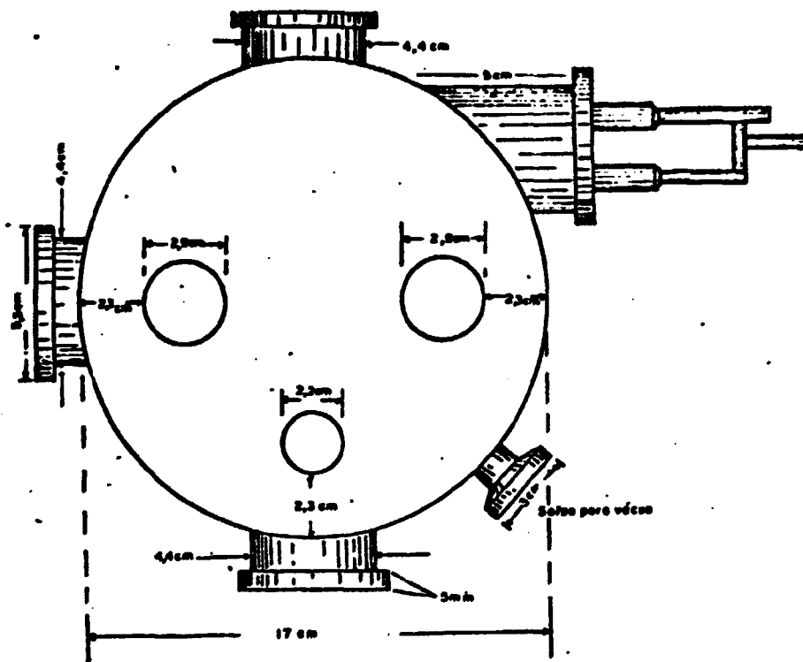
FIG. 3 VISTA DE BAIXO DA CÂMARA
