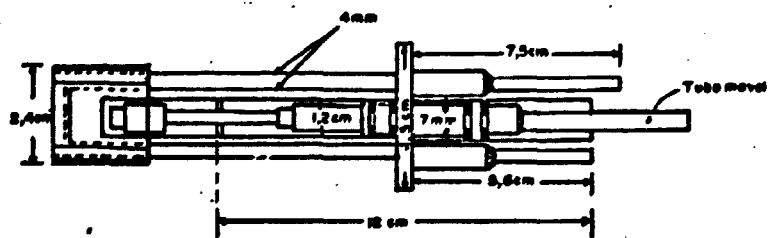
FIG. 4 PEÇA PARA APLICAÇÃO DA PRESSÃO
