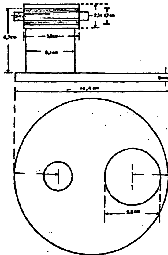
FIG. 2 TAMPA DA CÂMARA
