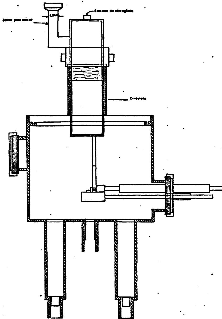
FIG. 1 CÂMARA COM CRIOSTATO
