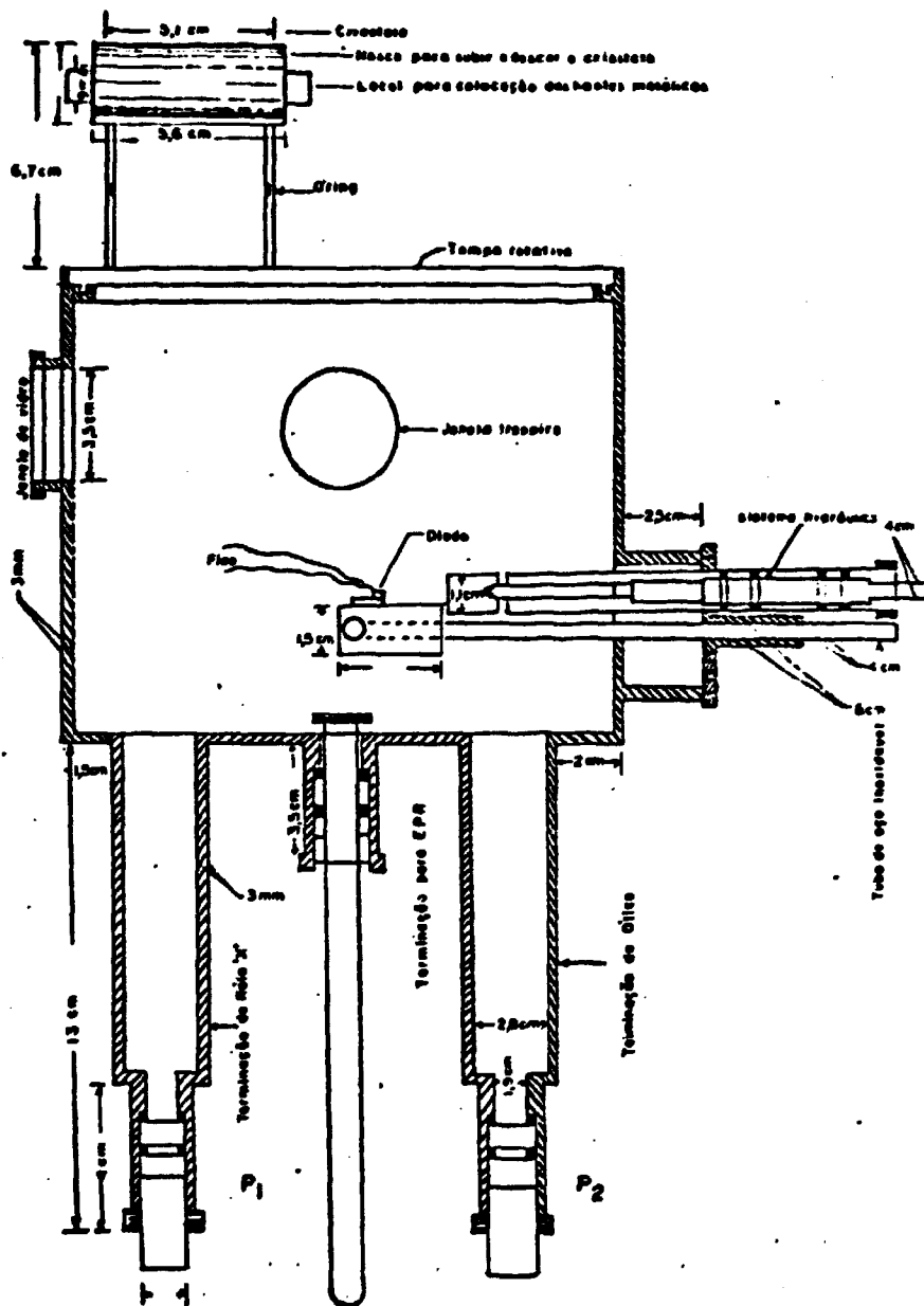
FIG. 5 CÂMARA PARA TROCA DE TERMINAÇÕES E APLICAÇÃO DE PRESSÃO UNIAXIAL A BAIXAS TEMPERATURAS
