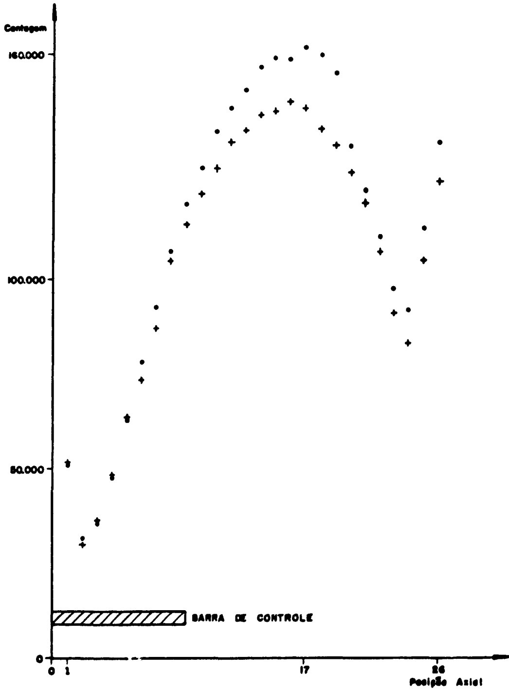
Figura 8 - Distribuição Axial do Elemento nº 101
