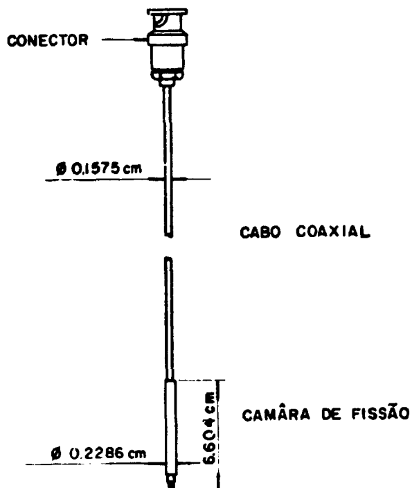
Figura 1 — Esquema da Câmara de Fissão Miniatura WL-23292
