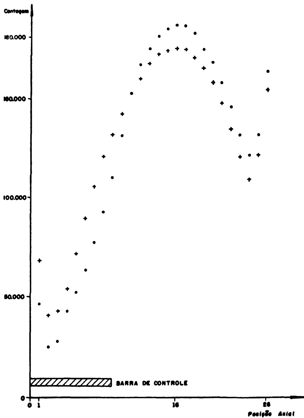
Figura 11 - Distribuição Axial do Elemento nº 108
