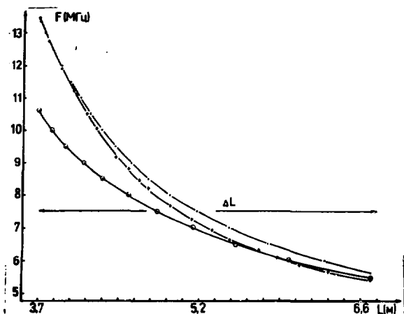
Рис. 3. \circ - частотный диапазон до модернизации, \bullet - частотный диапазон после модернизации /расчет/, + - частотный диапазон после модернизации /эксперимент/, \Delta L - диапазон движения закорачивающих пластин.
