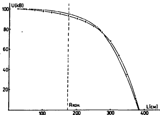
Рис. 5. • - для резонатора со старой геометрией на частоте 10,2 МГц, + - для модернизированного варианта резонатора на частоте 13,3 МГц. R_{\text{кон}} - конечный радиус ускорения.
