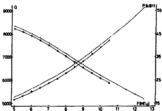
Рис. 4. \bullet - зависимость P=P(F) для резонатора со старой геометрией, \circ - зависимость P=P(F) для модернизированного резонатора, \bullet - зависимость Q=f(F) для резонатора со старой геометрией, + - зависимость Q=f(F) для модернизированного резонатора.
