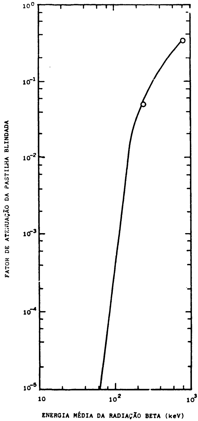
Figura 2 – Relação entre as respostas termoluminescentes das pastilhas blindadas e não blindadas em função da energia média da radiação beta.
