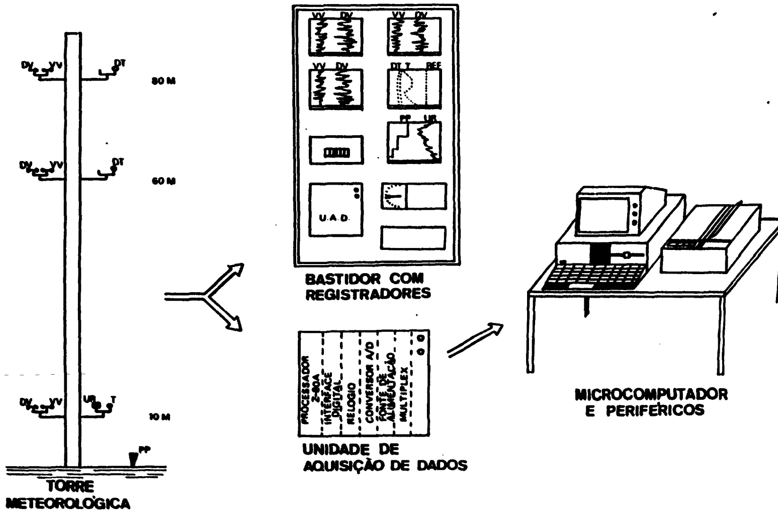
Figura 1. Esquema Simplificado do Sistema de Monitoração Meteorológica Desenvolvido pelo IPEN/COPESP.
