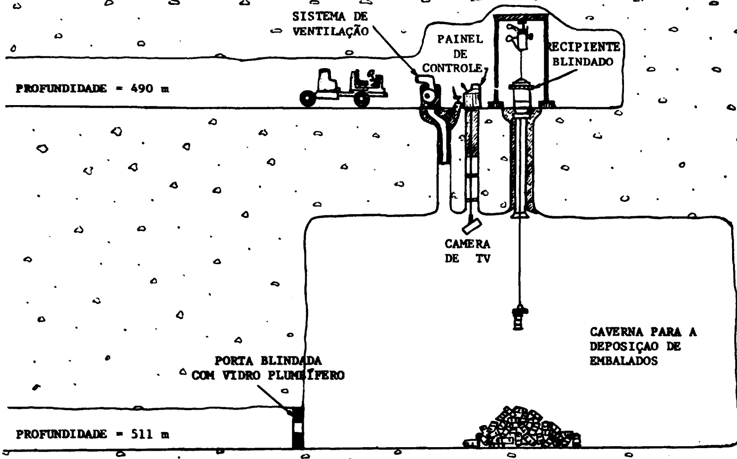
Figura 2 - Sistema de deposição de rejeitos radioativos, em mina de sal desativada, em Asse-Alemanha Oc, (6)
