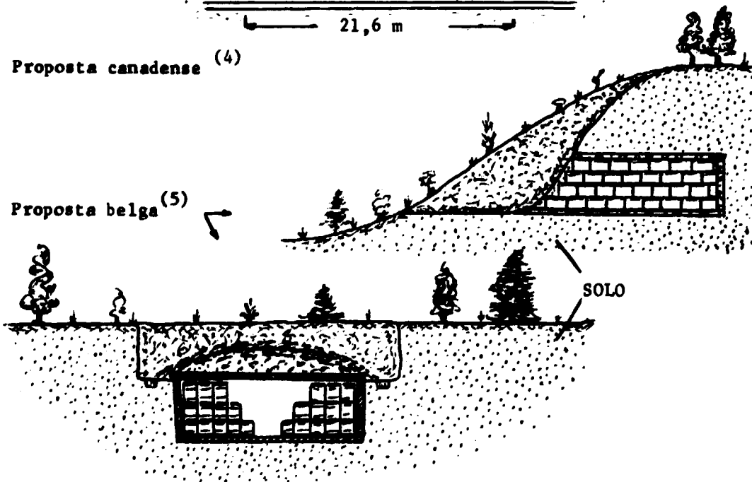
Figura 1 - Exemplos de deposição de rejeitos radioativos em locais pouco profundos da superfície.
