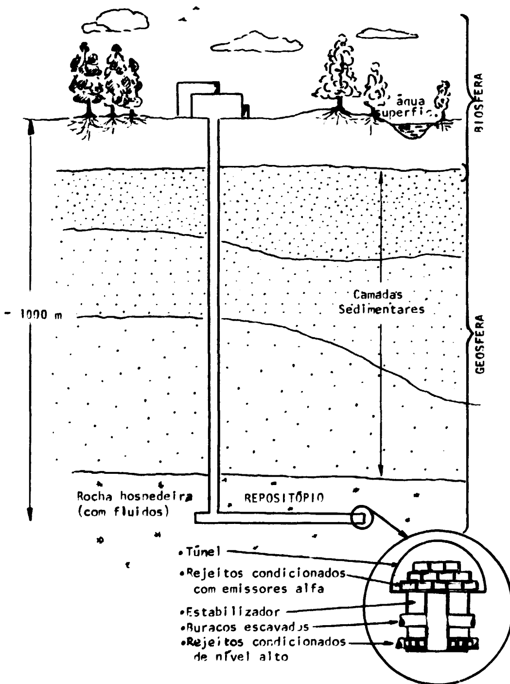
Figura 3 - Esquema de um sistema para deposição de rejeitos de nível alto.
