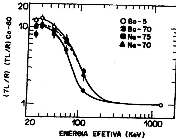
Figura 2. Curva de dependência energética das pastilhas normalizadas no Co-60.
