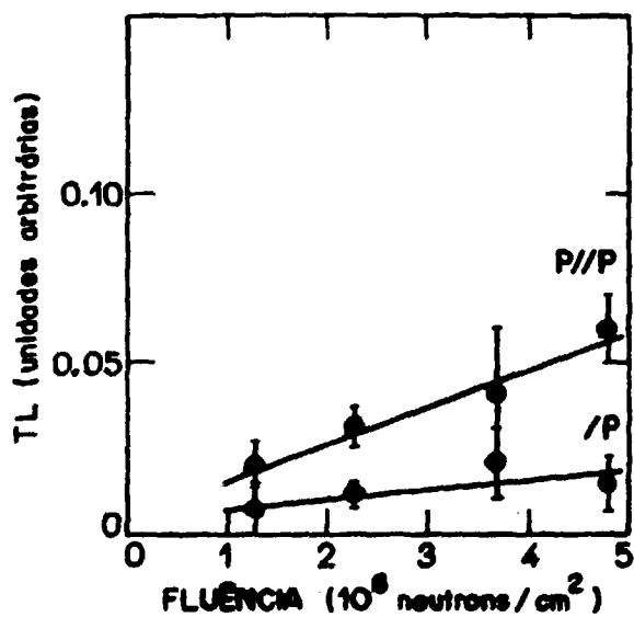
Figura 4. Resposta TL das pastilhas de \text{Na}_2\text{B}_4\text{O}_7 em função da fluência de nêutrons (P//P:parafina/fósforo/parafina e P/fósforo/parafina)
