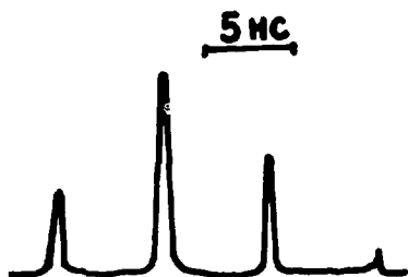
Рис. 2. Характерная форма цуга импульсов излучения генератора.
