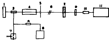
Рис. 1. Оптическая схема генератора /пояснения в тексте/.
