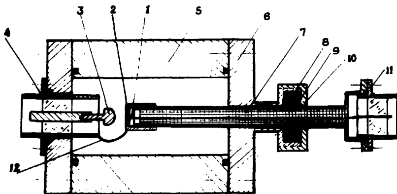
Рис. 3. Общий вид разрядника /пояснения в тексте/.
