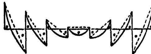
FIG. 2b: CASO 1 - TAB. 1, TUBO. GUIA (36)
