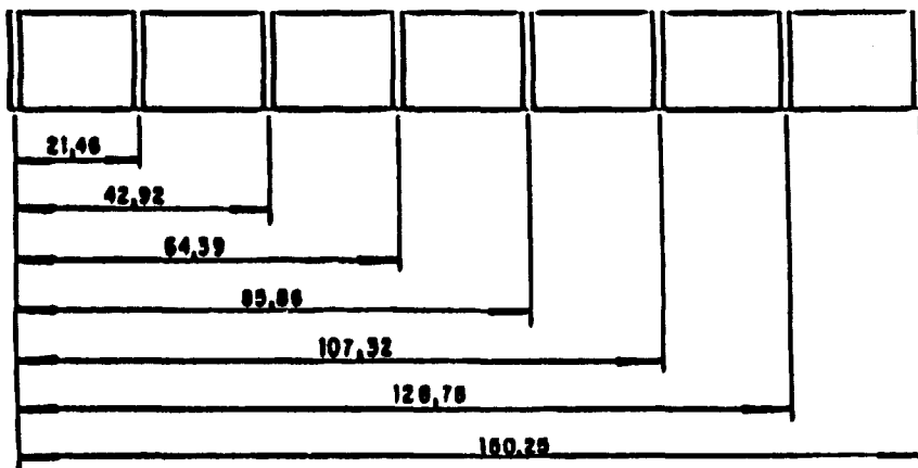
FIG. 1c: POSIÇÃO DAS GRADES ESPAÇADORAS
