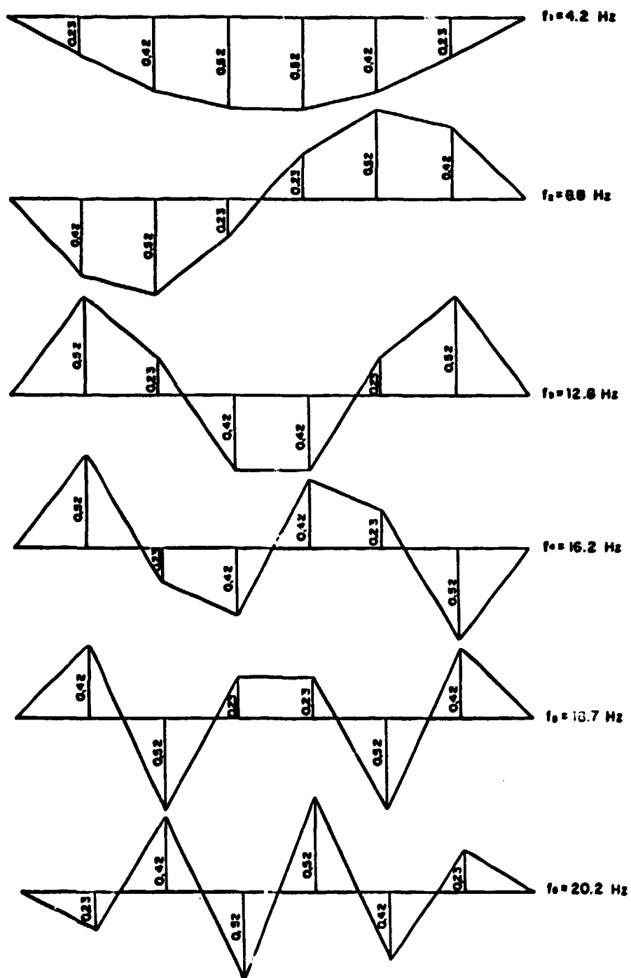
FIG. 5: MODOS DE VIBRAÇÃO DA ESTRUTURA INTEGRADA - CALCULADO COM ELCOM.
