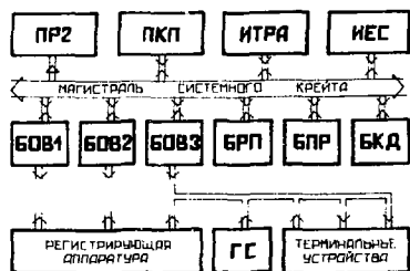
Рис.5. Блок-схема системы сбора данных: БКД - контроллер системного крейта; БПР - блок приоритетов; БРП - ручной контроллер; БОВ1 ÷ БОВ3 - интерфейсы ветви КАМАК; ПР2 - программируемый трековый процессор; ПКП - процессор для чтения и кодирования информации с ПК; ИТРА - интерфейс ЭВМ ТРА-1001i; ИЕС - интерфейс ЭВМ ЕС-1040; ГС - графическая система "Тектроникс 4051".
