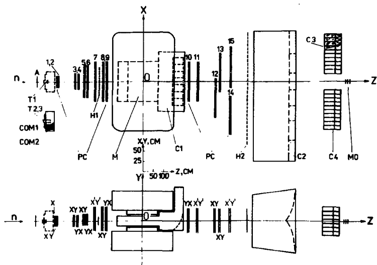
Рис. 2. Блок-схема спектрометра BIS-2: А - счетчик антисовпадений, T1÷T3 - мишени, COM1÷COM2 - детектор частиц отдачи, PC1÷15 - пропорциональные камеры, М - спектрометрический магнит, C1÷C2 - пороговые черенковские счетчики, H1÷H2 - сцинтилляционные годоскопы, C3÷C4 - ливневые черенковские счетчики, MO - нейтронный монитор.
