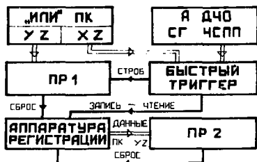
Рис. 4. Блок-схема системы отбора событий.
