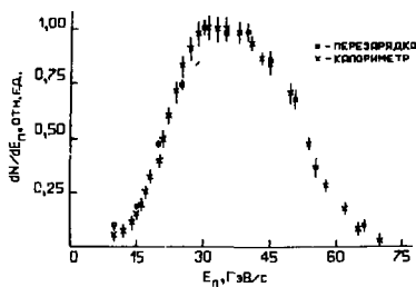
Рис. 1. Энергетический спектр нейтронов в канале 4N серпуховского ускорителя.
