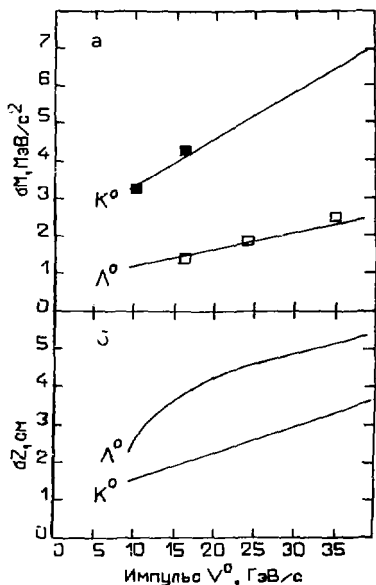
Рис. 6. Разрешение по эффективной массе (6а) и z-координате точки распада (6б) нейтральных каонов и \Lambda -гиперонов в зависимости от их импульса: линии - результаты расчета, точки - экспериментальные данные.
