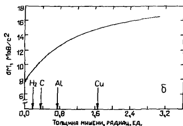
Рис. 8. Разрешения по эффективной массе для очарованного бариона \Lambda_C^+ в зависимости от его импульса для мод распада с участием K_S^0 -мезона (8а - верхняя кривая) и \Lambda -гиперона (8а - нижняя кривая) и толщины мишени (8б).
