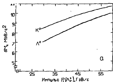
Рис. 8. Разрешения по эффективной массе для очарованного бариона \Lambda_C^+ в зависимости от его импульса для мод распада с участием K_S^0 -мезона (8а - верхняя кривая) и \Lambda -гиперона (8а - нижняя кривая) и толщины мишени (8б).
