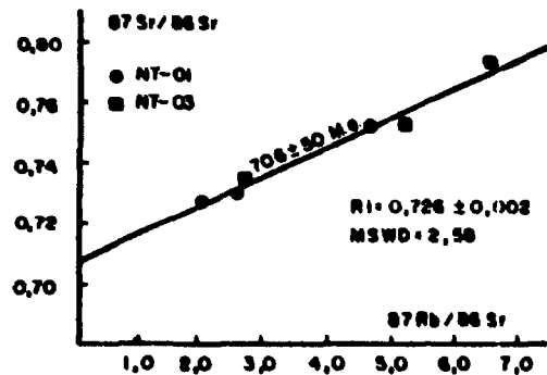
FIGURA 2c - ISÓCRONA Rb/Sr EM ROCHA TOTAL DE GNAISSES DA REGIÃO DE ABUTÃ
