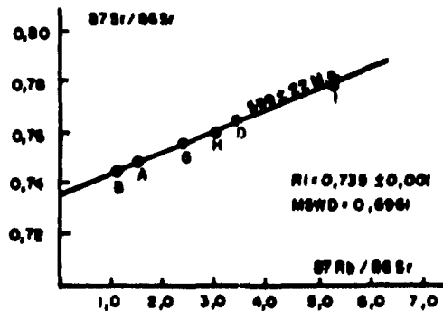
FIGURA 2b - ISÓCRONA Rb/Sr EM BIOTITA MISTOS, NOVA TRENTO (S.C.)
