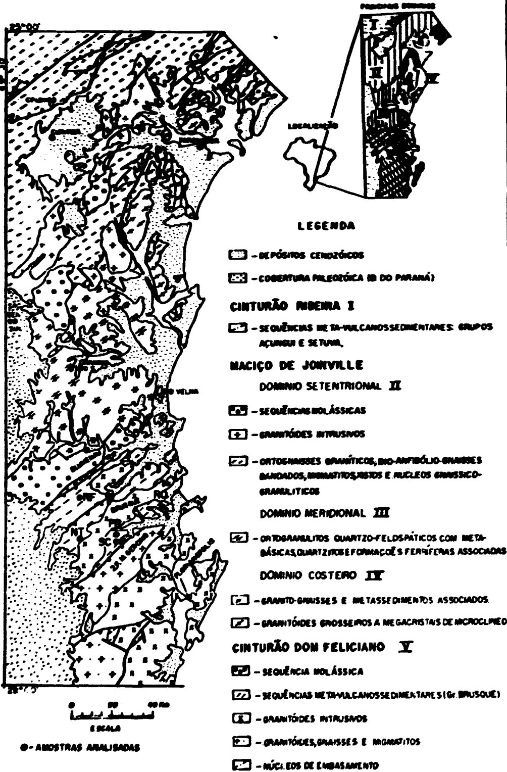
FIG. 1 - O GRUPO BRUSQUE NO CONTEXTO GEOTECTÔNICO DOS ESTADOS DO PARANÁ E SANTA CATARINA
