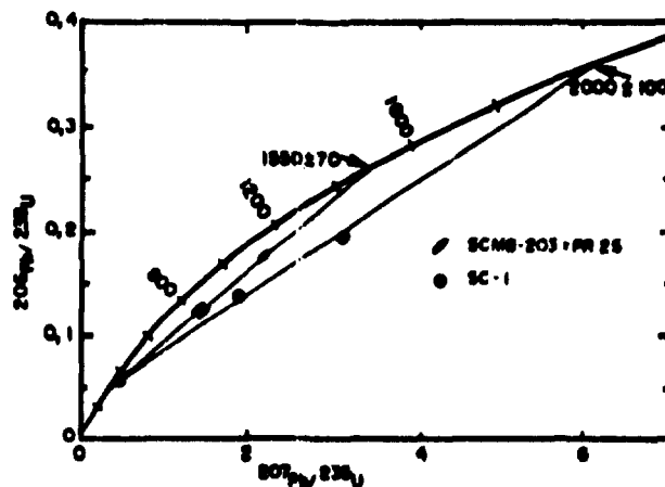
FIGURA 2d - DADOS U-Pb EM ZIRCÕES DE DUAS AMOSTRAS DO GRUPO BRUSQUE SC.
