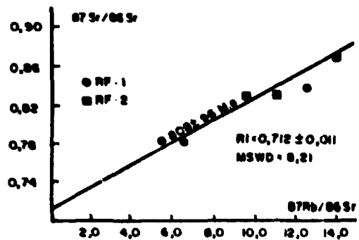
FIGURA 2a - ISÓCRONA Rb/Sr EM FILITOS DO RIBEIRÃO DO RUSSO (BOTUVERÁ)
