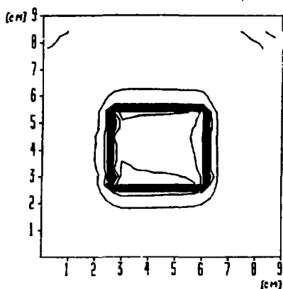
Рис. 3. Примеры изодозных распределений протонных пучков с энергиями 200, 100 и 130 МэВ (а, б, в) и поперечных изоуровней узких протонных пучков (г, д), полученных с помощью изодозографа с миниатюрным кремниевым детектором 116 .
