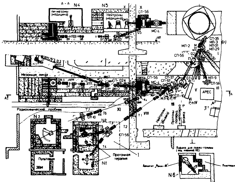
Рис. 1. Схема каналов медицинских пучков и расположение процедурных кабин на фазотроне ОИЯИ.
