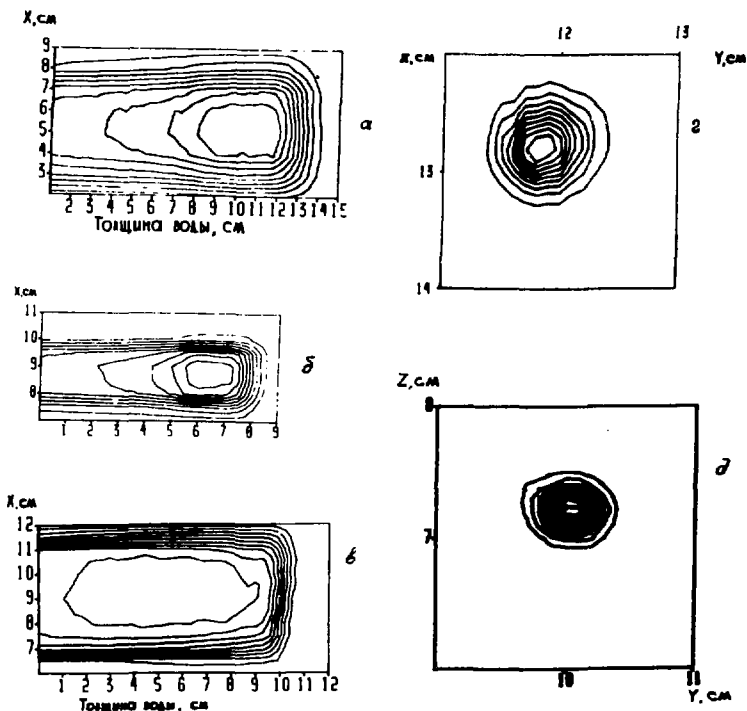
Рис. 3. Примеры изодозных распределений протонных пучков с энергиями 200, 100 и 130 МэВ (а, б, в) и поперечных изоуровней узких протонных пучков (г, д), полученных с помощью изодозографа с миниатюрным кремниевым детектором 116 .
