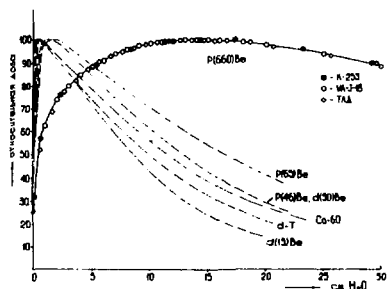
Рис. 6. Изоурвни поперечного сечения мезонного пучка в фокусе широкоугольной магнитной линзы, полученные с помощью изодозографа с кремниевым детектором 16/ .
