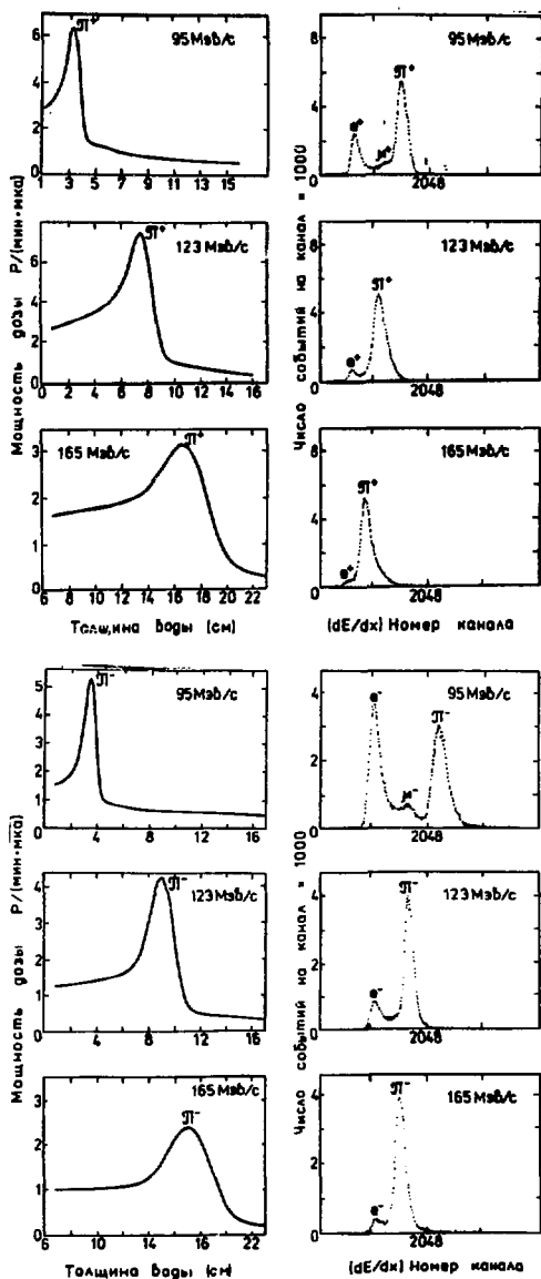
Рис. 4. Примеры глубинных дозных распределений мезонных пучков и dE/dx -спектров, полученных с помощью изодозографа и сцинтилляционных счетчиков.
