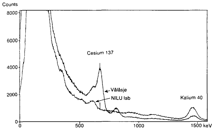
Figur 11: Bakgrunnspektrum fra stasjon 756 Vålåsjø sammenlignet med et spektrum opptatt på NILU.
