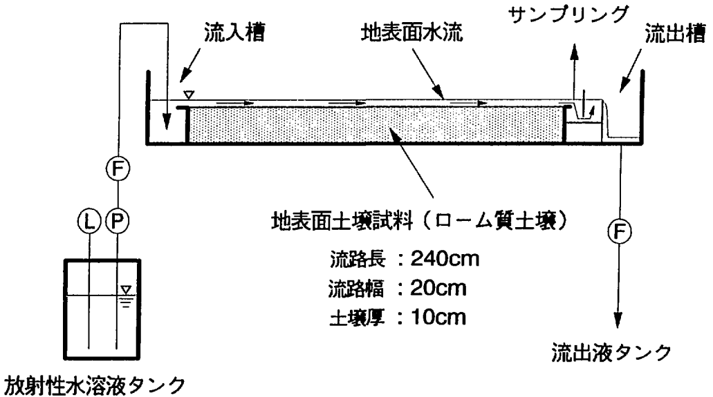
図2 試験装置および試験方法の概略
