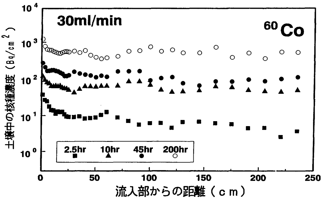
図6-1 流下方向の土壌中核種濃度分布
