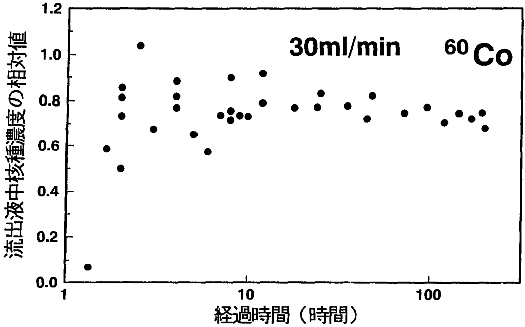
図5-1 流出液中核種濃度の経時変化
