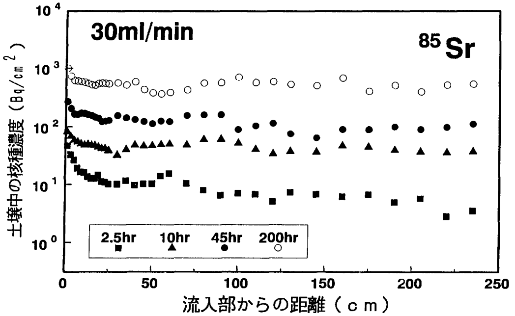
図6-2 流下方向の土壌中核種濃度分布
