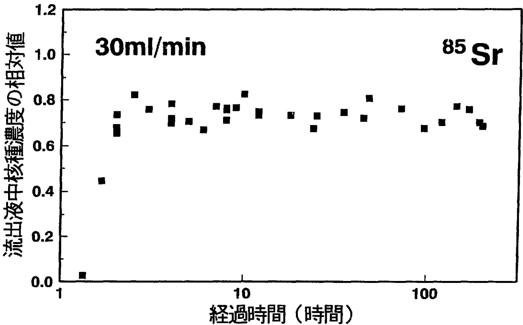
図5-2 流出液中核種濃度の経時変化
