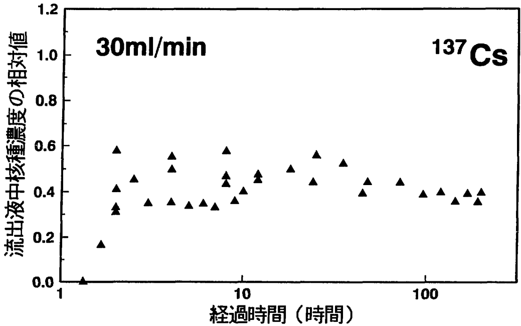
図5-3 流出液中核種濃度の経時変化
