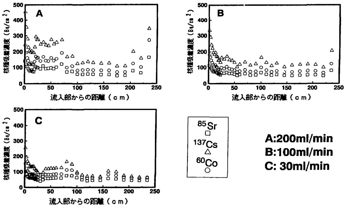
図4 流下方向の土壤中核種濃度分布
