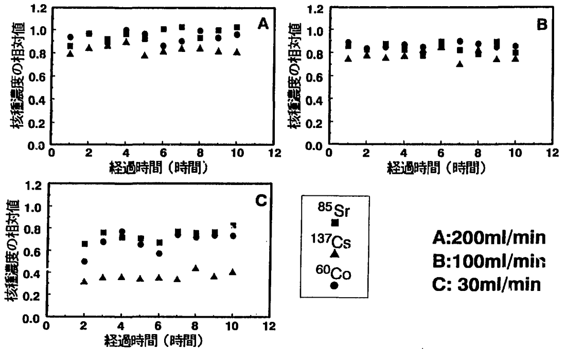
図3 流出液中核種濃度の経時変化
