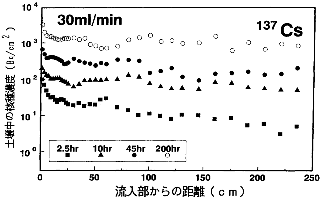
図6-3 流下方向の土壌中核種濃度分布
