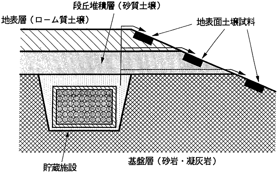
図1 想定される核種の移行経路
