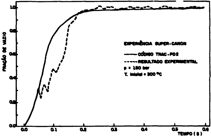
FIG:4- Evolução da fração de vazio. Abertura total do tubo (100mm).
