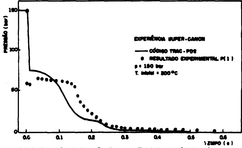
FIG:5- Evolução da Pressão. Abertura Total do tubo (100mm).
