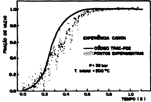
Fig:2 - Evolução da fração de vazio. Abertura total do tubo (100mm).
