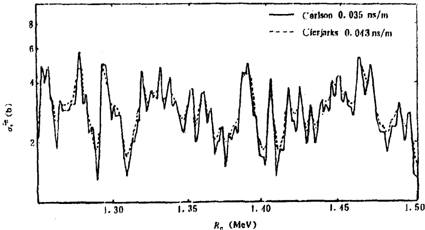
图5 Carlson 与 Cierjarks \sigma_t^{\text{Fe}} 测量值的比较(1~1.5MeV)
