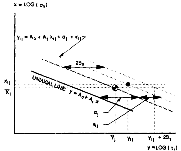
FIG. 13 STATISTICAL MODEL PARAMETERS
