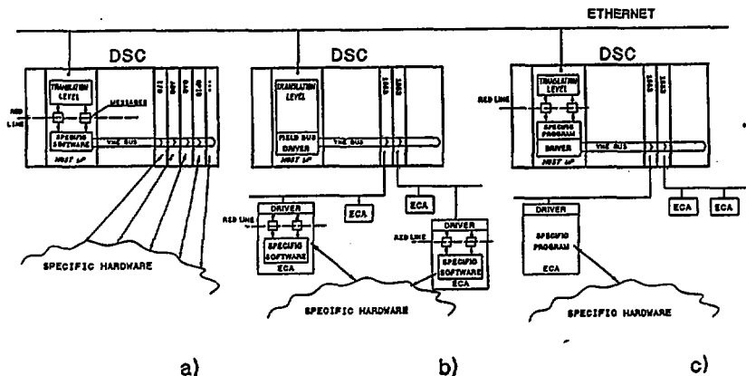
Figure 3. Actual implementation schemes
