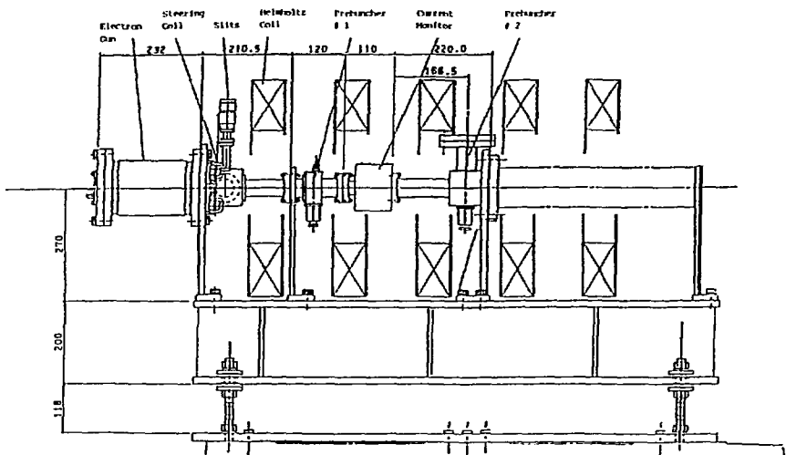
図2. 新入射器
