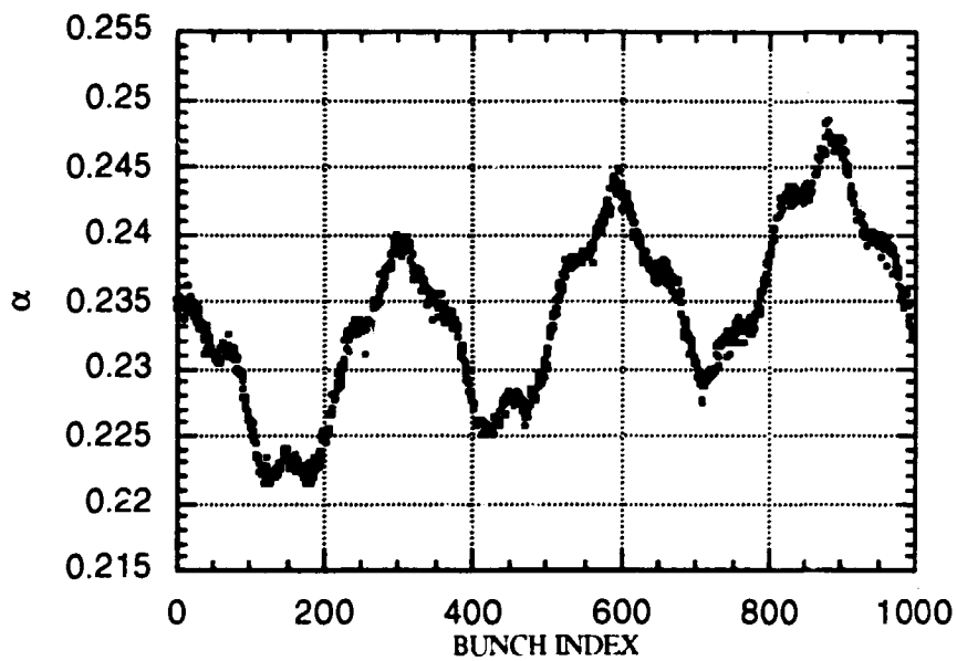
Figure 15: Twiss parameter \alpha
