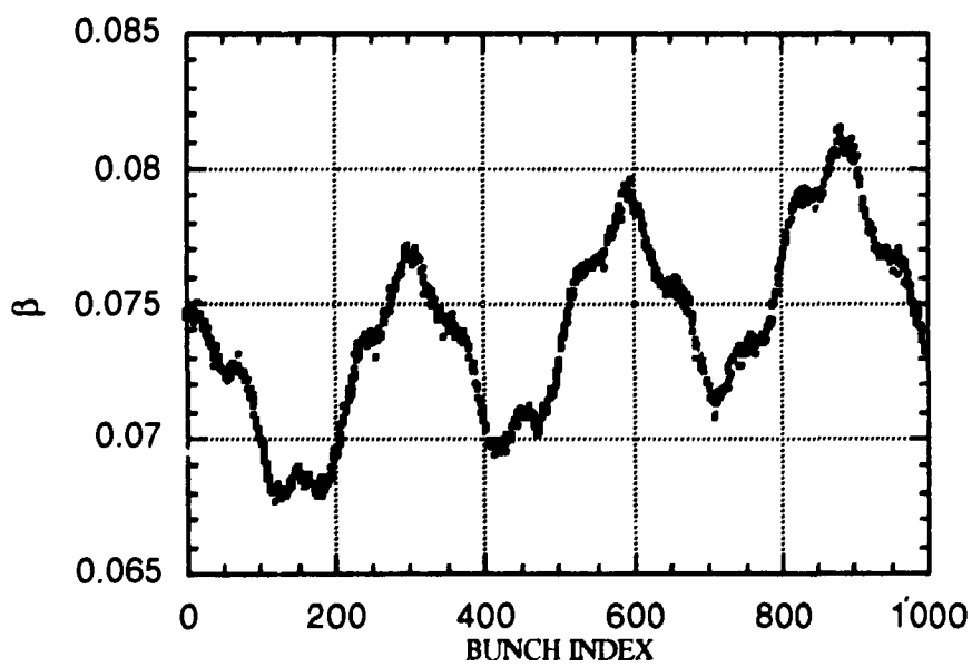
Figure 16: Twiss parameter \beta
