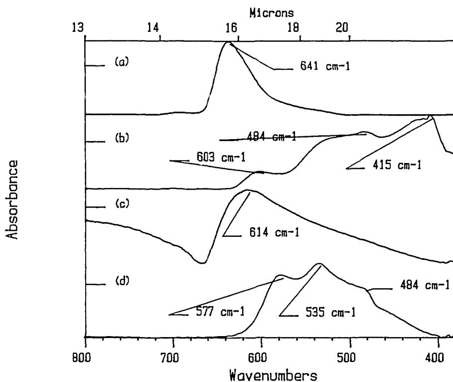
Figur 1. FTIR-spektra från ett Pt-förslutet kvartsprovör (a) och från den läckande Pt-förslutningen (b). Figurena (c) och (d) visar spektra från \text{Cu}_2\text{O} i KBr respektive \text{CuO} i KBr.
