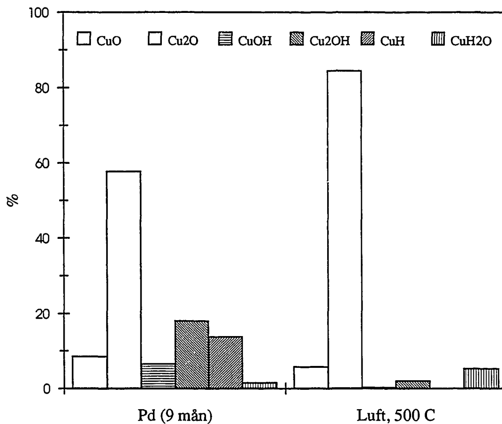
Figur 5. Distribution av olika Cu-O-H fragment vid SIMS-analys av oxidationsprodukter på koppar i Pd-förslutet system vid 50 °C och i luft vid 500 °C
