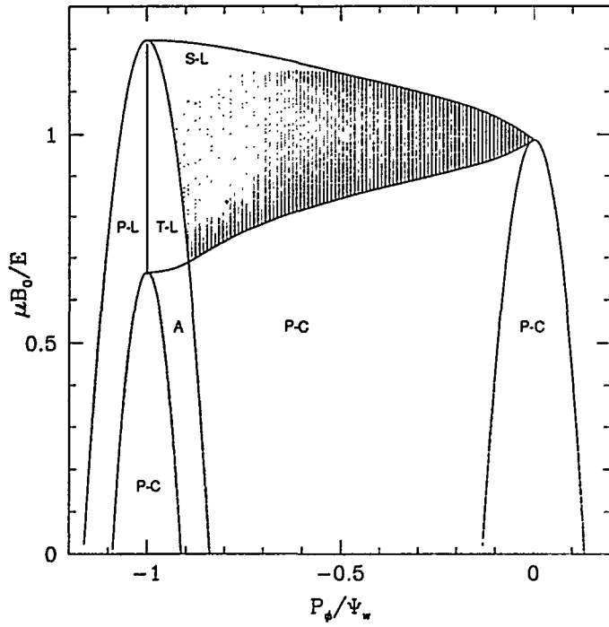
Fig. 25. Confinement domain, 100 keV, equilibrium 67885.
