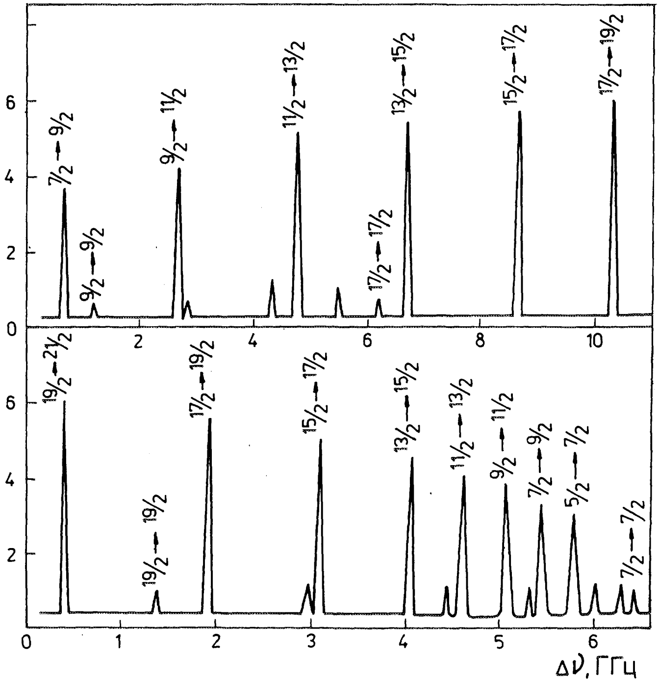
Рис. 2. Спектр резонансной лазерной флуоресценции для перехода с \lambda=591,5 нм между основным ^5L^0 и возбужденным ^7M_7 состояниями ^{233}\text{U} (вверху) и ^{235}\text{U} (внизу)
