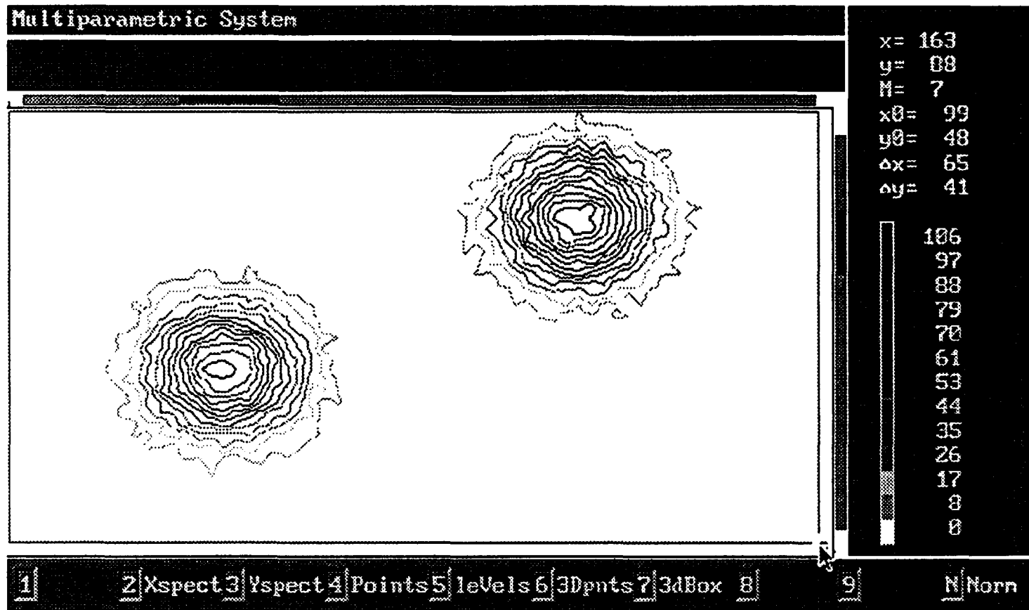
Fig.2 Espectro de coincidencias \gamma - \gamma del radioisótopo ^{99}\text{Mo} . Detalle de dos picos con curvas de nivel
