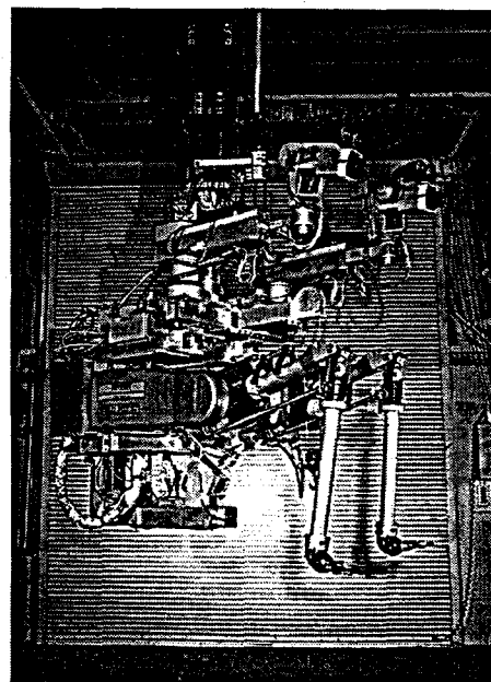
Fig. 2. M2 servomanipulator
