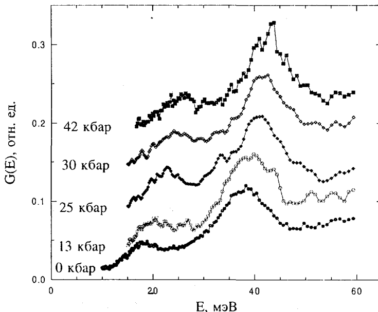
Рис.10 Обобщенная плотность колебательных состояний для образца \text{NH}_4\text{Br}
