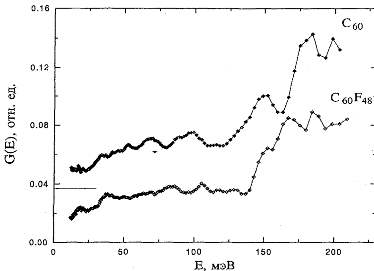
Рис. 11. Обобщенная плотность колебательных состояний для образцов фуллерена C_{60} и фулерида C_{60}F_{48}
