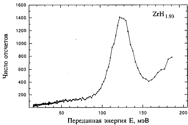
Рис. 5. Спектр неупругого рассеяния на образце ZrH_{1.93}
