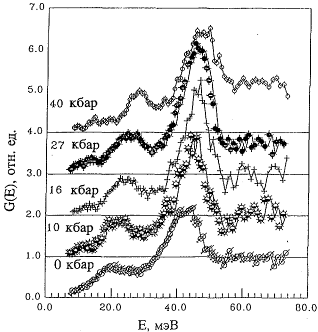
Рис.9. Обобщенная плотность колебательных состояний для образца NH_4Cl
