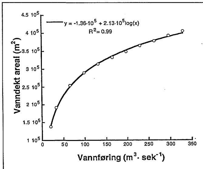
Figur 8. Vanndekt areal ( m^2 ) ved ulike vannføringer ( m^3 \text{ sek}^{-1} ) for området mellom kraftverksutløpet og Harestrømmen (4 km). Linjen angir en logaritmisk regresjon.
