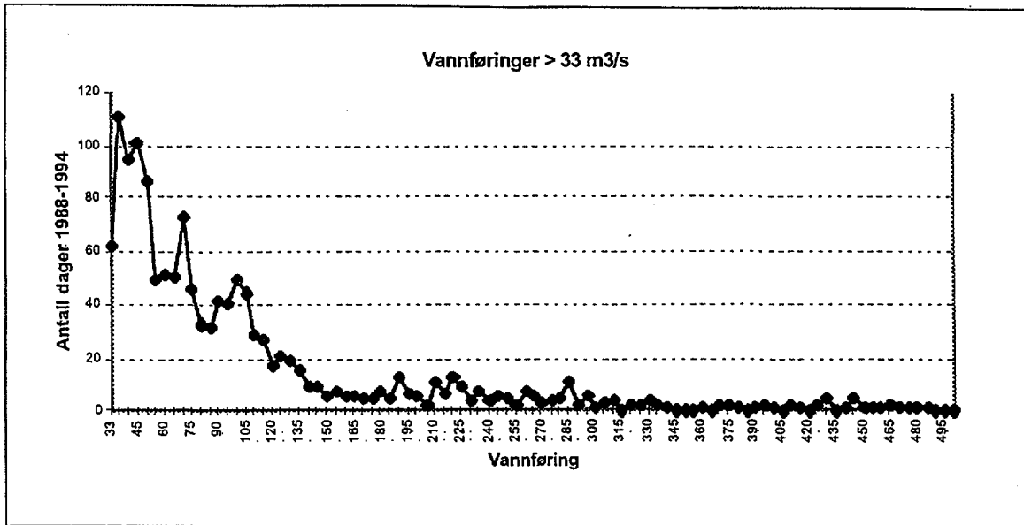
Figur 7. Frekvens (antall dager) av ulike vannføringer ( m^3 \text{ sek}^{-1} ) i Altaelva ved Kista i perioden 1988-94. Dager med vannføring mindre enn 33 m^3 \text{ sek}^{-1} er ikke tatt med i figuren, dvs. 1178 dager (46,1 %) i syvårs perioden. 20 dager med vannføringer større enn 500 m^3 \text{ sek}^{-1} er heller ikke inkludert.
