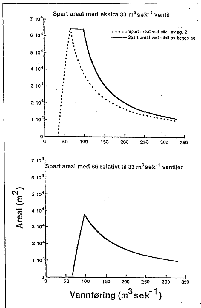
Figur 10. Areal mellom kraftverkutløpet og Harestrømmen som unngår tørlegging ved ulike typer utfall dersom det monteres en ekstra 33 \text{ m}^3 \text{ sek}^{-1} forbitappings-ventil, og ekstra besparelse dersom det i stedet monteres en 66 \text{ m}^3 \text{ sek}^{-1} ventil.
