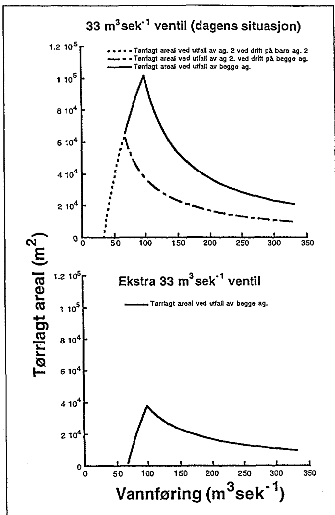
Figur 9. Tørrlagt areal ( m^2 ) i området mellom kraftverkutløpet og Harestrømmen (ca 4 km) ved ulike vannføringer ( m^3 \text{ sek}^{-1} ) er gitt for ulike typer utfall med dagens forbitappingsventil og en ekstra 33 \text{ m}^3 \text{ sek}^{-1} ventil. Ved en ekstra 66 \text{ m}^3 \text{ sek}^{-1} ventil vil alle utfall kunne kompenseres.
