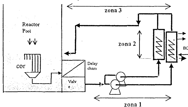
Gambar 4. Pembagian Zona Heat Loss Pendingin Primer
