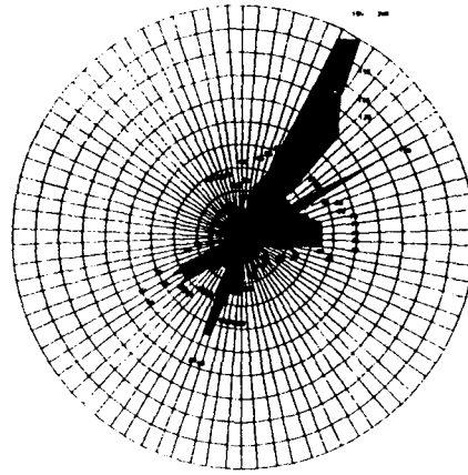
Фиг.2 "Роза" на ветровете
