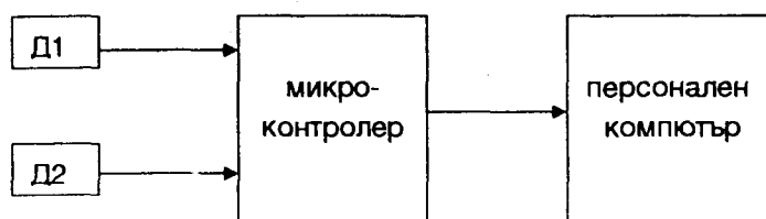
Фиг. 1. Блокова схема на компютъризирана система за построяване "розата" на ветровете, определяне скоростта и средната плътност на мощността на вятъра.
