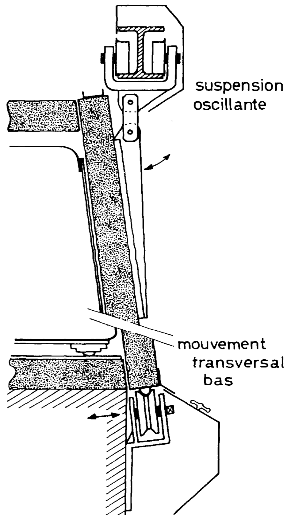
Fig. 12. _ CHAINE "CASTOR" MOUVEMENTS des PORTES BLINDEES
