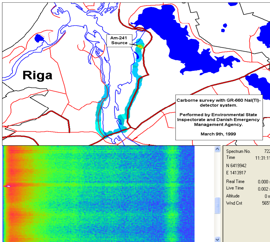
Figur 2.3. Ved rekognisering med en lettisk målebil (leveret i forbindelse med øststøtteprogrammet) gav gammaspæktrometret et kraftigt udslag ved passage af en byggetomt (hvid prik til venstre i serien af spektre). Det viste sig at være en ameri-cium-kilde.
