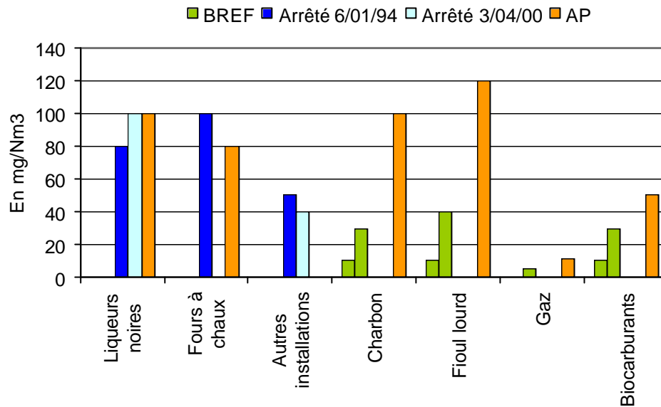
Figure 7. Valeurs d'émission pour les poussières des fours des installations de production de pâte à papier, de papier et de carton (en fonction du combustible utilisé)
