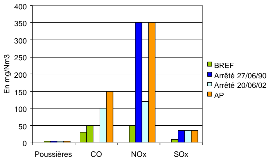
Figure 2. Valeurs d'émission pour les rejets atmosphériques des nouvelles grandes installations de combustion brûlant du gaz naturel
