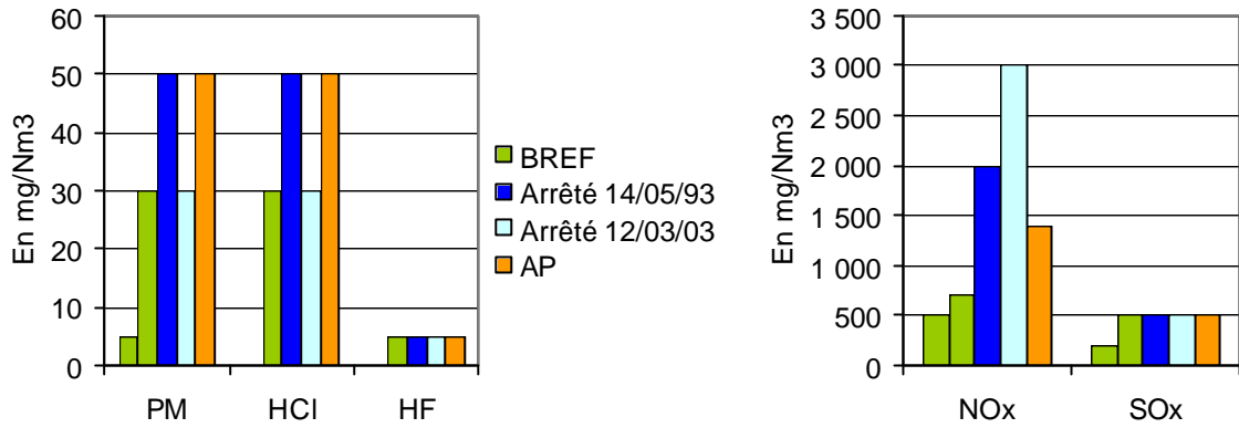
Figure 4. Valeurs d'émission pour les rejets atmosphériques des verreries (verres non spéciaux, fours brûlant du gaz)
