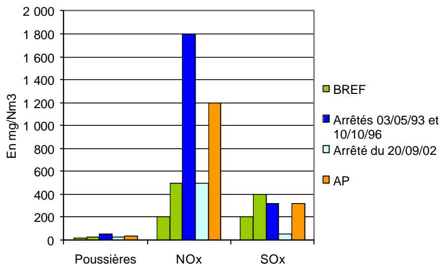
Figure 3. Valeurs d'émission pour les rejets atmosphériques des nouvelles cimenteries co-incinérant des déchets spéciaux
