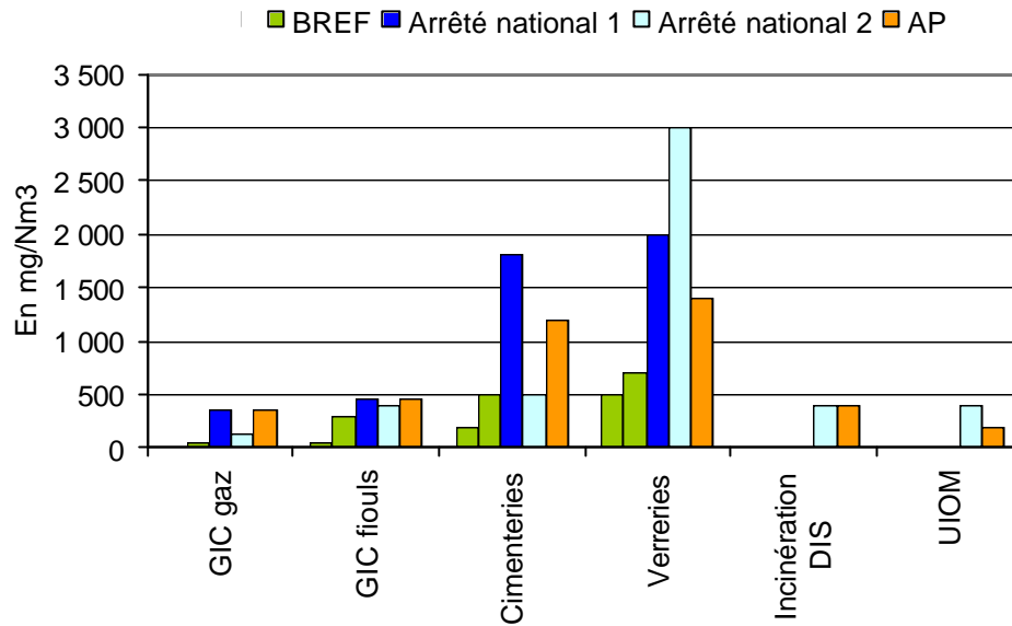
Figure 12. Valeurs d'émission pour les rejets d'oxydes d'azote, pour différents secteurs
