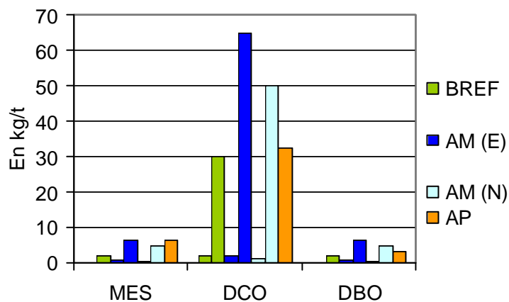
Figure 8. Valeurs d'émission pour les rejets aqueux d'installations de production de pâte à papier nouvelles (N) et existantes (E) 23 avec utilisation de vieux papiers
