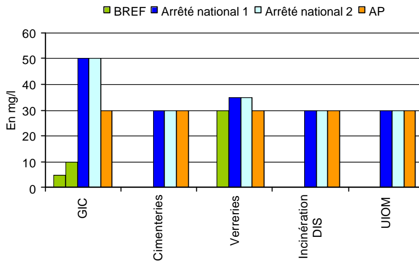
Figure 14. Valeurs d'émission pour les rejets de matières en suspension (MES), pour différents secteurs
