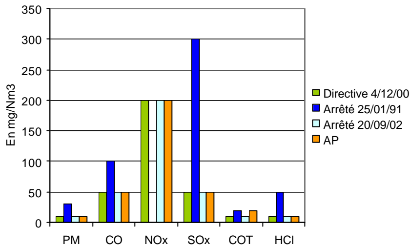
Figure 6. Valeurs d'émission pour les rejets atmosphériques des installations d'incinération de déchets municipaux 20
