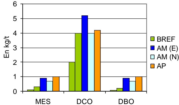
Figure 9. Valeurs d'émission pour les rejets aqueux d'installations de production de pâte à papier nouvelles (N) et existantes (E) 24 sans utilisation de vieux papiers
