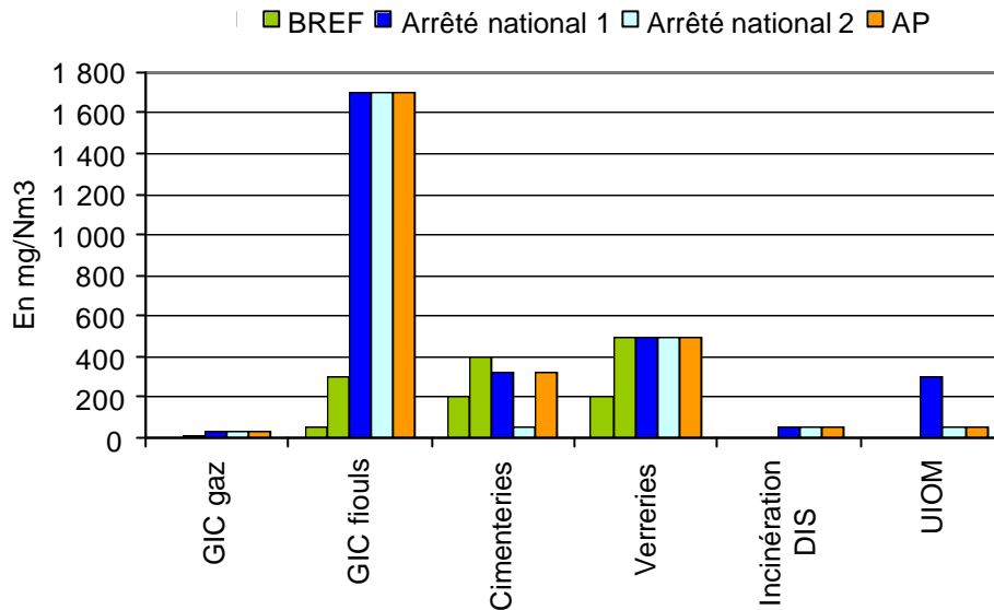
Figure 13. Valeurs d'émission pour les rejets d'oxydes de soufre, pour différents secteurs
