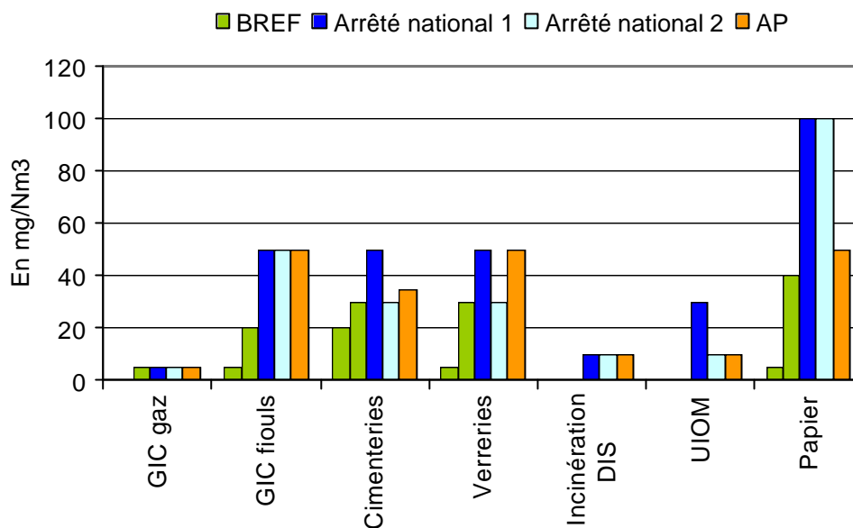
Figure 11. Valeurs d'émission pour les rejets de poussière, pour différents secteurs
