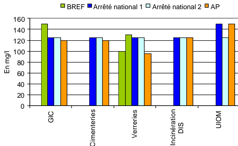
Figure 15. Valeurs d'émission pour la demande chimique en oxygène (DCO), pour différents secteurs
