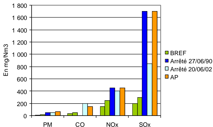
Figure 1. Valeurs d'émission pour les rejets atmosphériques des nouvelles grandes installations de combustion brûlant des combustibles liquides, de puissance thermique comprise entre 50 et 100 MW
