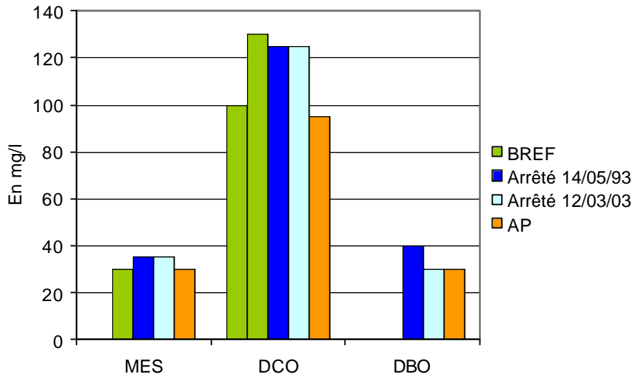
Figure 5. Valeurs d'émission pour les rejets d'eaux résiduaires dans le milieu naturel pour les verreries
