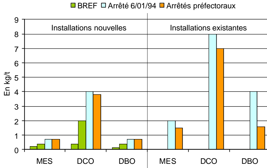
Figure 10. Valeurs d'émission pour les rejets aqueux des installations, nouvelles et existantes, de production de papier et carton
