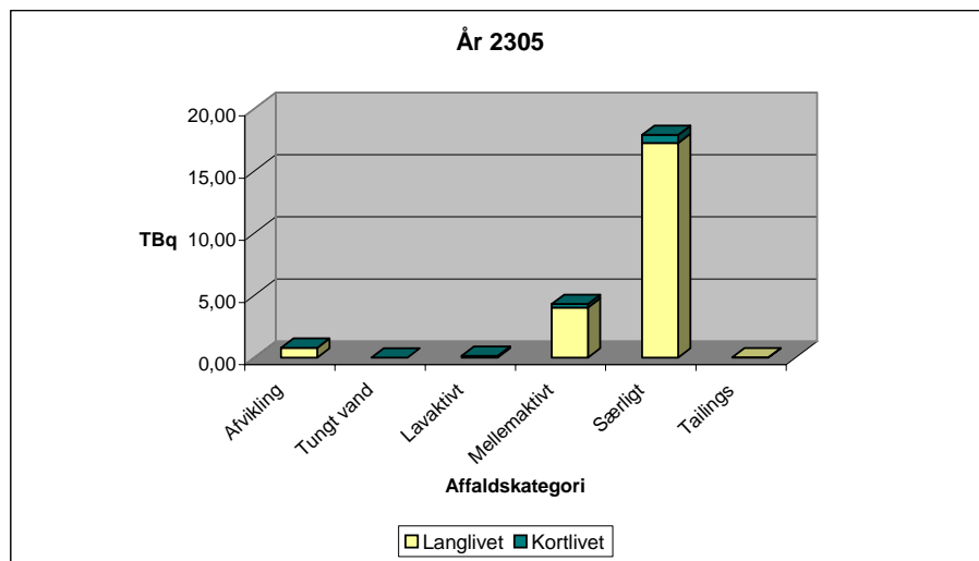
Figur 3.1: Henfald i aktivitet i dansk radioaktivt affald
