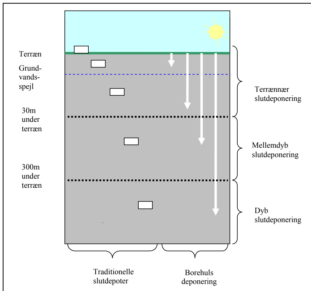
Figur 6.1: Vertikal placering af slutdepot
