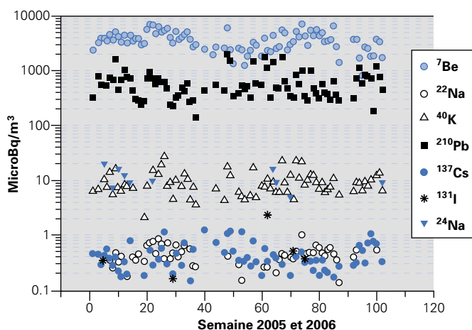
Figure 3 : Concentrations radioactives mesurées dans l'air à l'aide du collecteur haut débit (700 \text{m}^3/\text{h} ) installé par l'OFSP sur le site de Meyrin.
