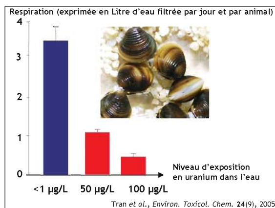
Figure 2 : Une faible concentration en uranium dans l'eau diminue le taux de respiration des animaux exposés (en rouge) d'un facteur 4-5 par rapport à celui d'organismes non exposés (en bleu).
