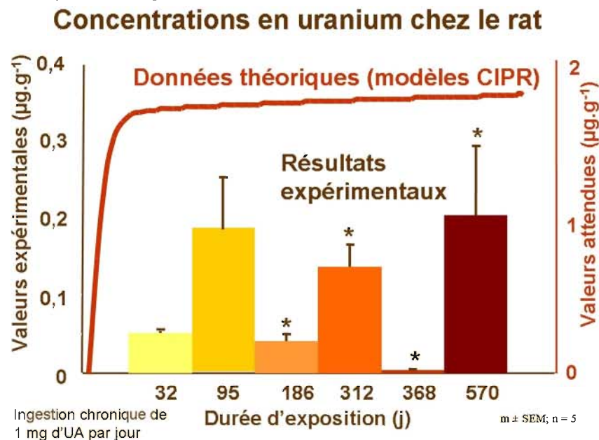
Figure 1. Concentration en uranium dans l'organisme du rat après ingestion chronique d'uranium appauvri (UA) via l'eau de boisson. Les résultats expérimentaux obtenus montrent, pour la plupart des tissus et organes analysés, des cinétiques particulières d'accumulation (histogramme), distinctes de celles prédites par les modèles usuels, qui extrapolent les données provenant de contaminations aiguës (courbe rouge).
